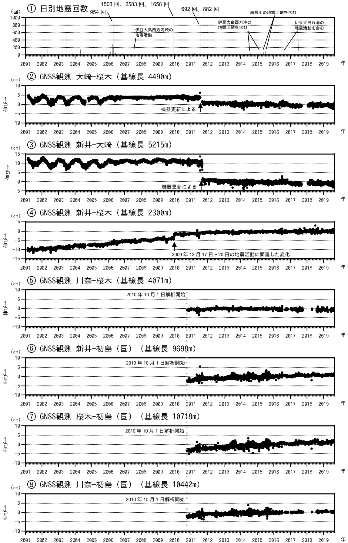
図3 伊豆東部火山群 火山活動経過図（2001年1月1日～2019年8月31日）
