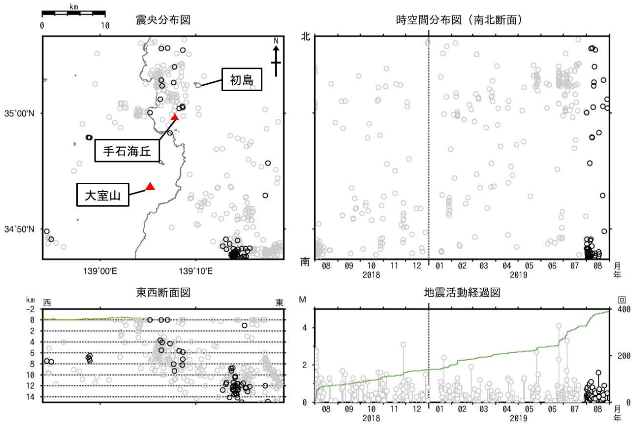
図2 伊豆東部火山群 広域地震観測網による震源分布図（2018年8月1日～2019年8月31日）
