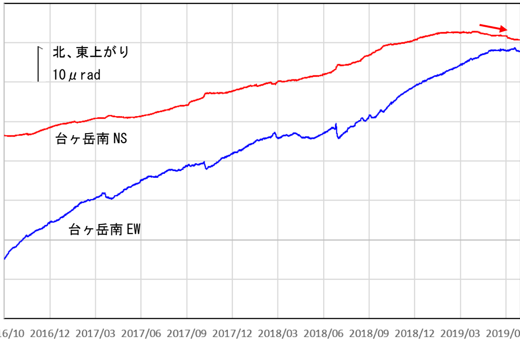
図6 箱根山 台ヶ岳南観測点における傾斜データ（2016年10月1日～2019年6月30日）
