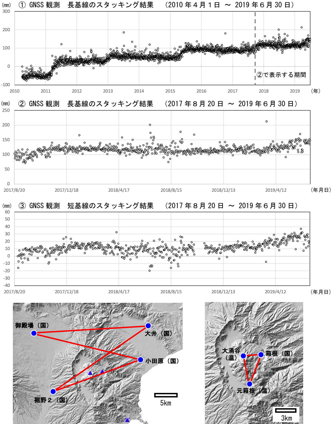
図9 スタッキング手法による箱根山のGNSS基線長変化 および 基線図 ①、②のスタッキングは左下の基線長の組み合わせ、③のスタッキングは右下の基線長の組み合わせを用いている。
