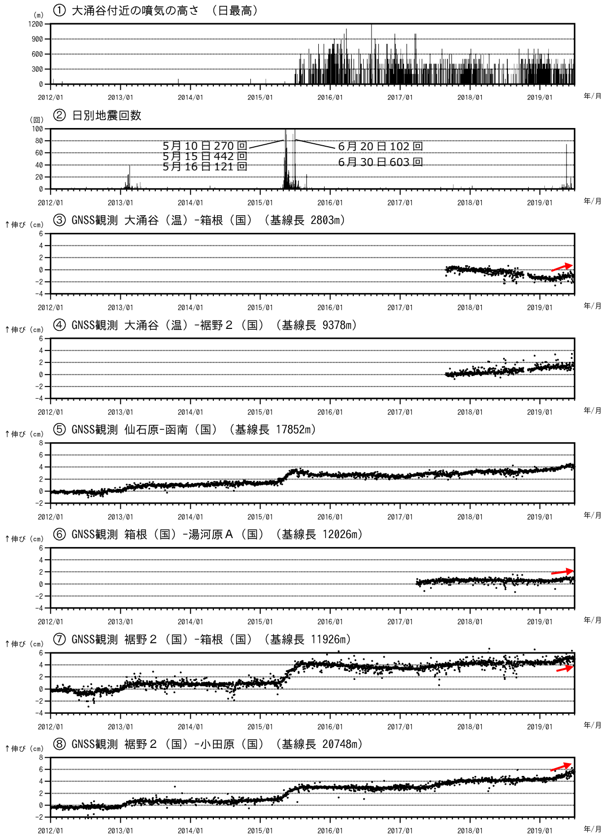
図7 箱根山 火山活動経過図（2012年1月1日～2019年6月30日）
