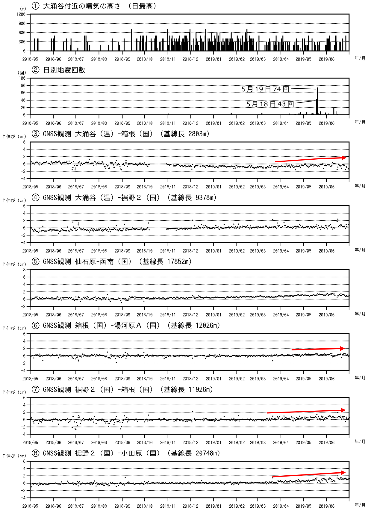
図8 箱根山 火山活動経過図（2018年5月1日～2019年6月30日）
