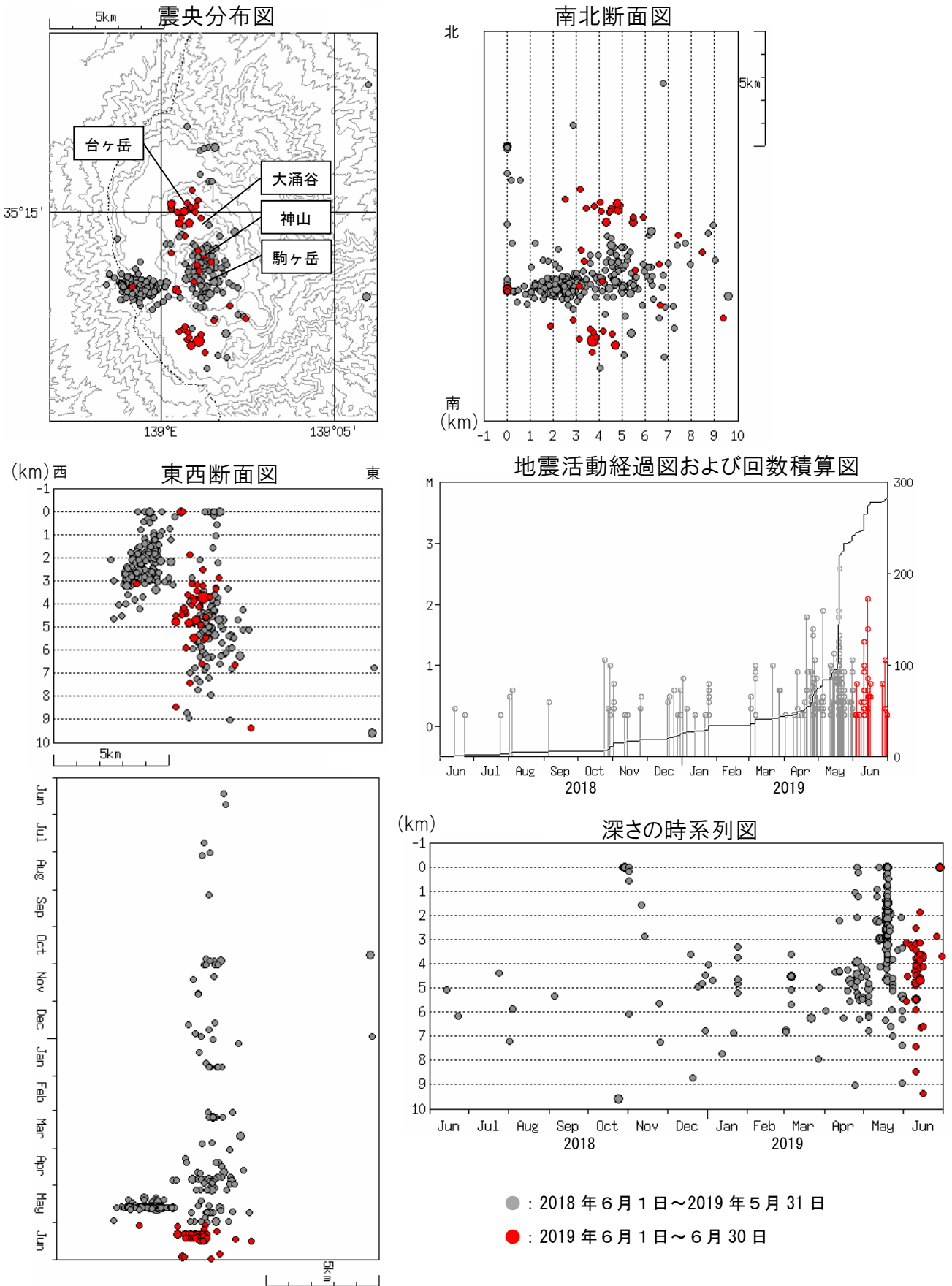
図10 箱根山 広域地震観測網による山体周辺の震源分布図(2018年6月1日～2019年6月30日)
