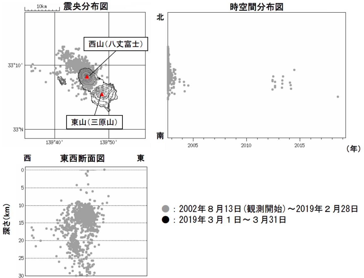
図3 八丈島 震源分布図（2002年8月13日～2019年3月31日） ・今期間、震源が求まる地震はありませんでした。
