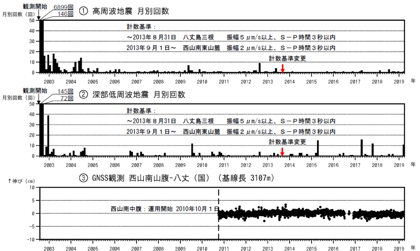
図2 八丈島 火山活動経過図(2002年8月13日~2019年3月31日)
