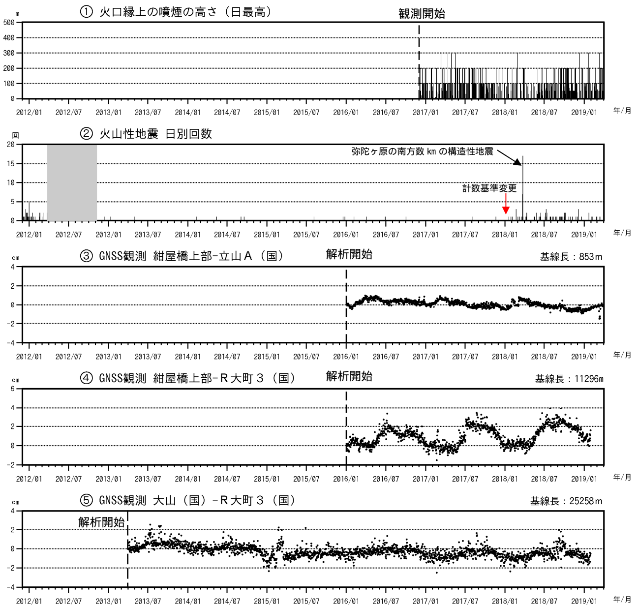
図 3 弥陀ヶ原 火山活動経過図（2011 年 12 月 1 日～2019 年 3 月 31 日）
