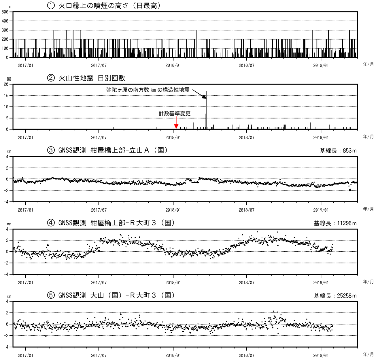
図4 弥陀ヶ原 最近の火山活動経過図(2016年12月1日~2019年3月31日)
