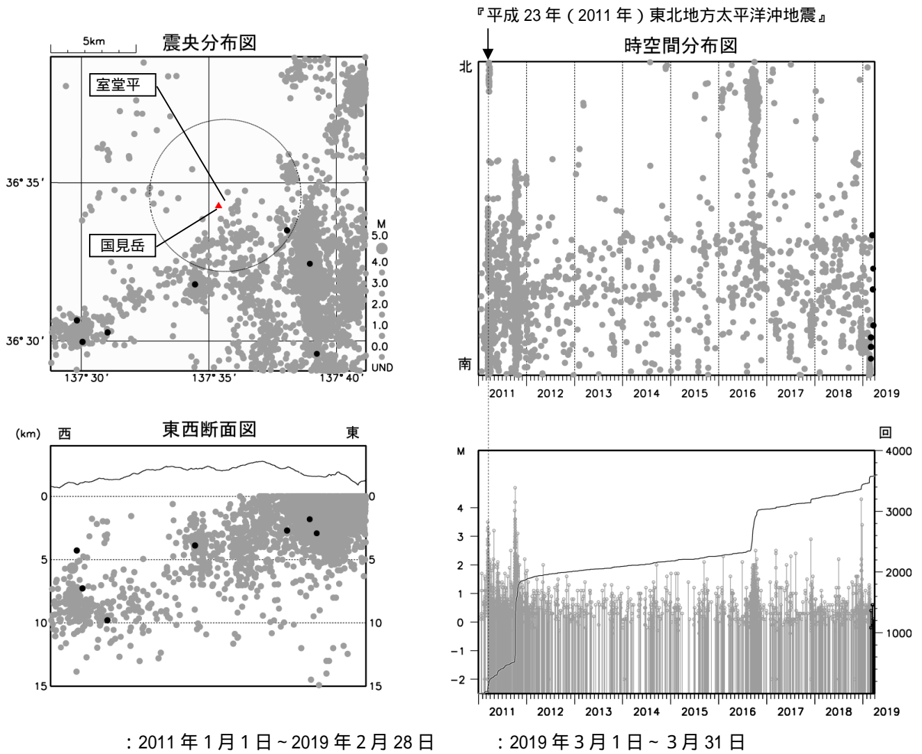
図2 弥陀ヶ原 広域地震観測網による山体・周辺の地震活動(2011年1月1日~2019年3月31日)
