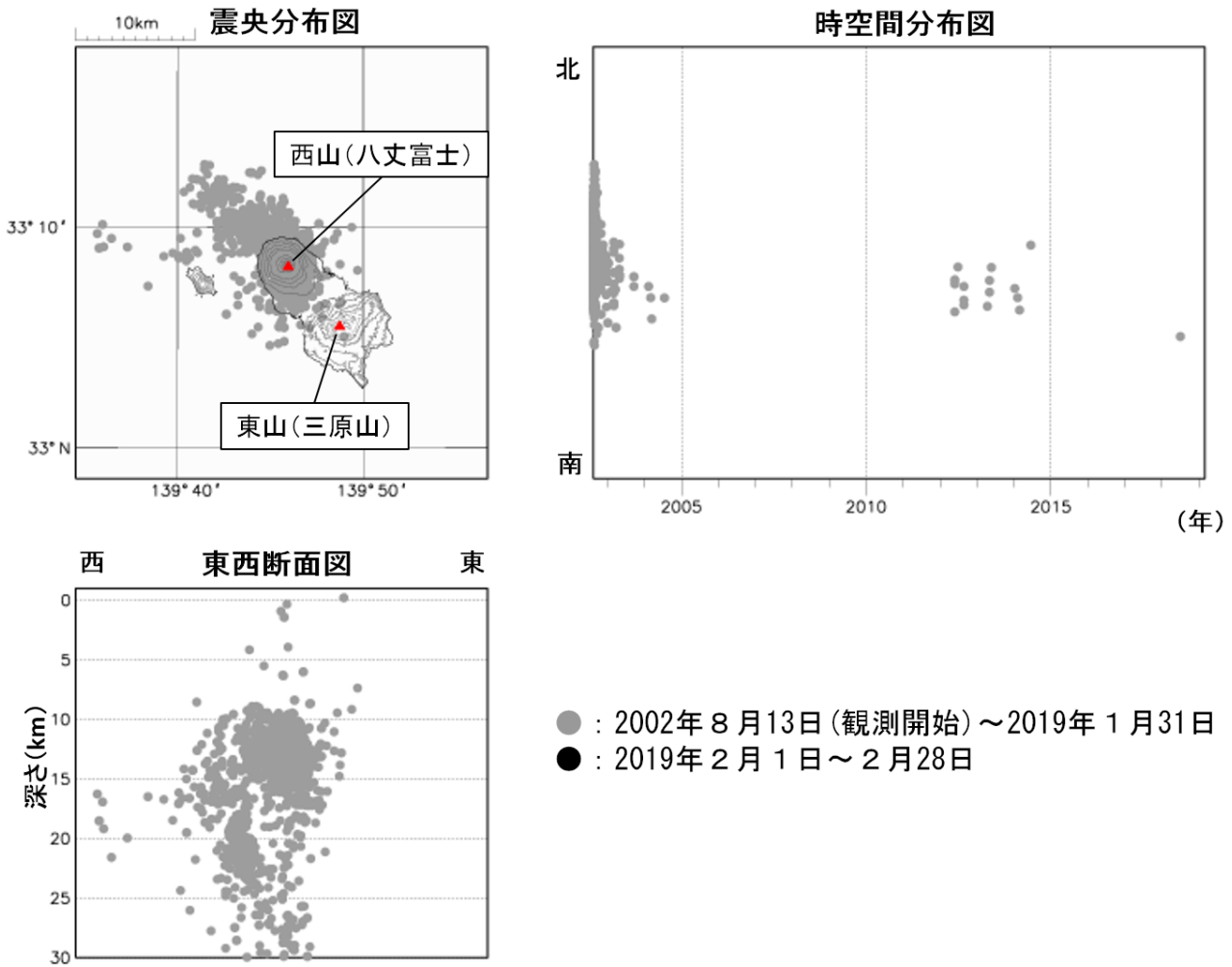
図3 八丈島 震源分布図 (2002年8月13日～2019年2月28日) ・今期間、震源が求まる地震はありませんでした。
