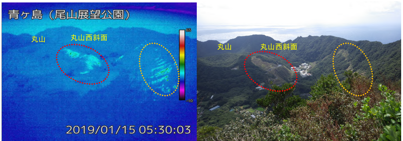
図2 青ヶ島 カルデラ内の地表面温度 2) の状況(左:1月15日 尾山展望公園監視カメラによる、右:2016年3月15日に撮影した同場所からの写真)
