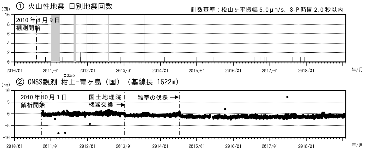
図3 青ヶ島 火山活動経過図(2010年8月9日~2019年1月31日) グラフの灰色部分は機器障害による欠測。 (国): 国土地理院、図4のGNSS基線 に対応。グラフの空白部分は欠測。
