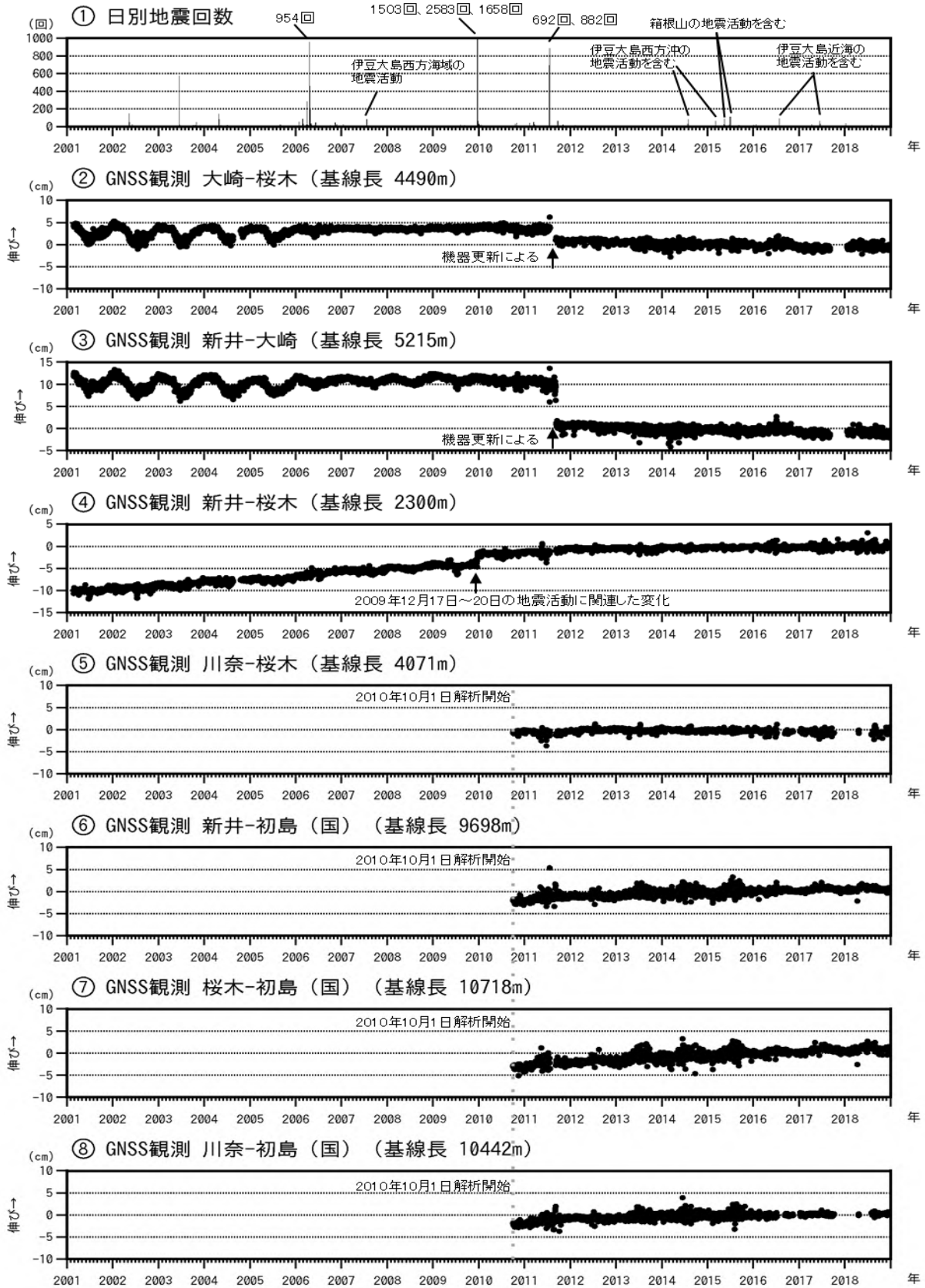
図3 伊豆東部火山群 火山活動経過図(2001年1月1日~2018年12月31日)
