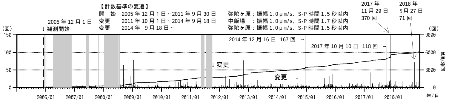
図 3 白山 地震活動経過図及び地震回数積算（2005 年 12 月 1 日 ~ 2018 年 11 月 30 日）
