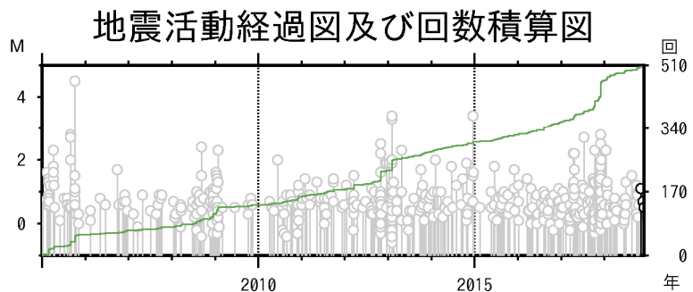
図 4 白山 広域地震観測網による山体・周辺の地震活動（2005 年 1 月 1 日 ~ 2018 年 11 月 30 日）
