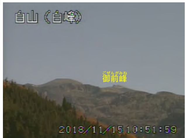
図 2 白山 山頂部の状況 （11 月 15 日 白峰監視カメラによる）
