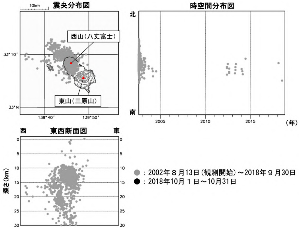
図3 八丈島 震源分布図(2002年8月13日~2018年10月31日) ・今期間、震源が求まる地震はありませんでした。
