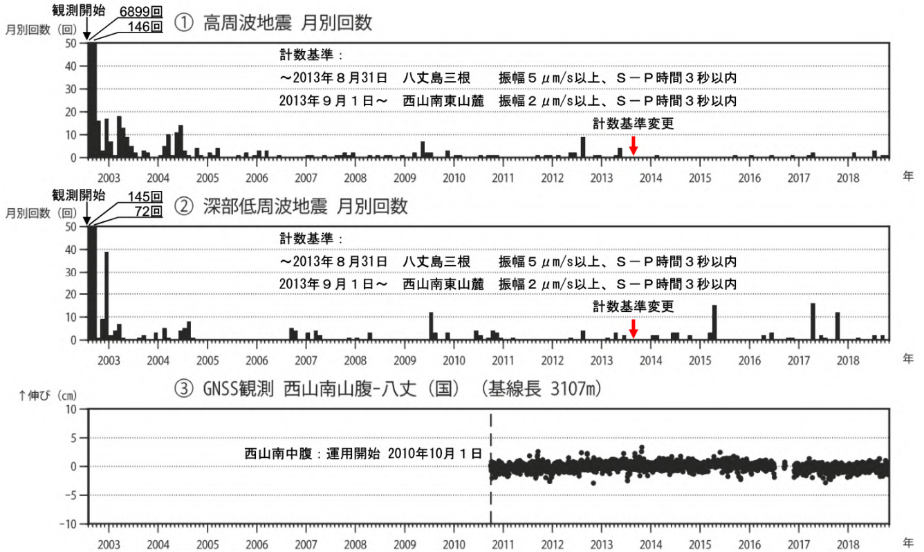
図2 八丈島 火山活動経過図(2002年8月13日~2018年10月31日)
