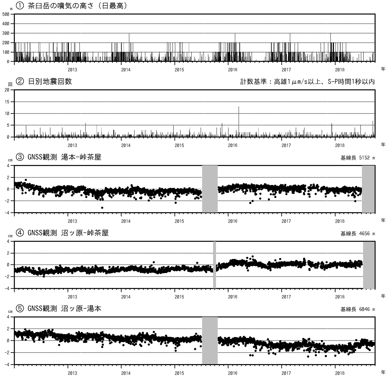
図4 那須岳 火山活動経過図(2012年1月1日~2018年9月30日)
