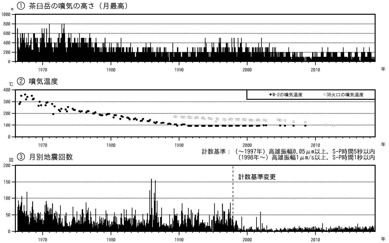
図 3 那須岳 火山活動経過図（1966 年 1 月～2018 年 9 月）
