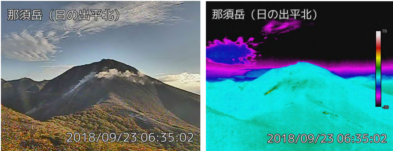
図 2 那須岳 茶臼岳の可視画像と赤外熱映像装置 1) による地表面温度分布(日の出北監視カメラによる)
