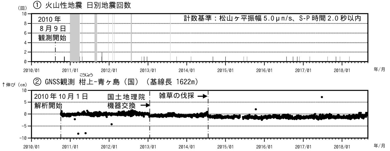
図2 青ヶ島 火山活動経過図（2010年8月9日～2018年8月31日） グラフの灰色部分は機器障害による欠測。 （国）：国土地理院、図3のGNSS基線 に対応。グラフの空白部分は欠測。
