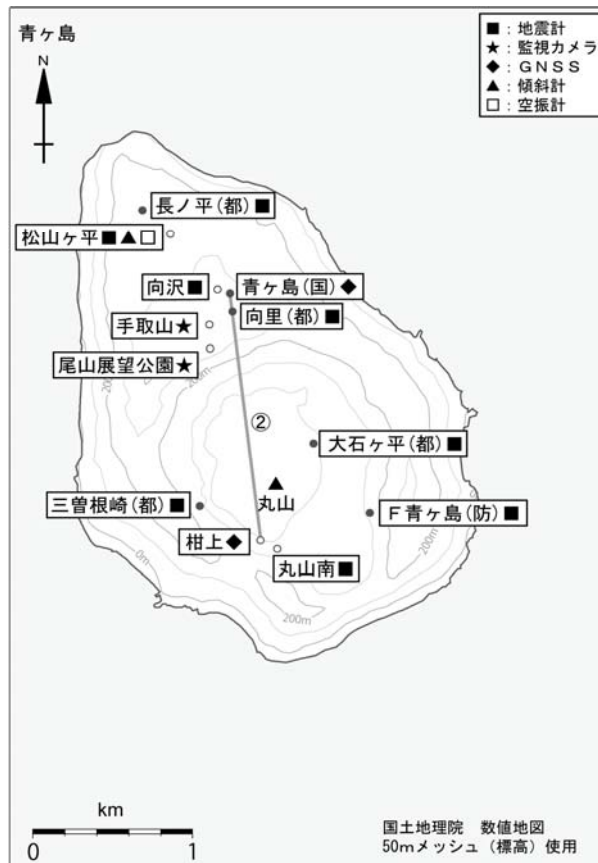
図3 青ヶ島 観測点配置図 GNSS基線は図2の②に対応しています。
