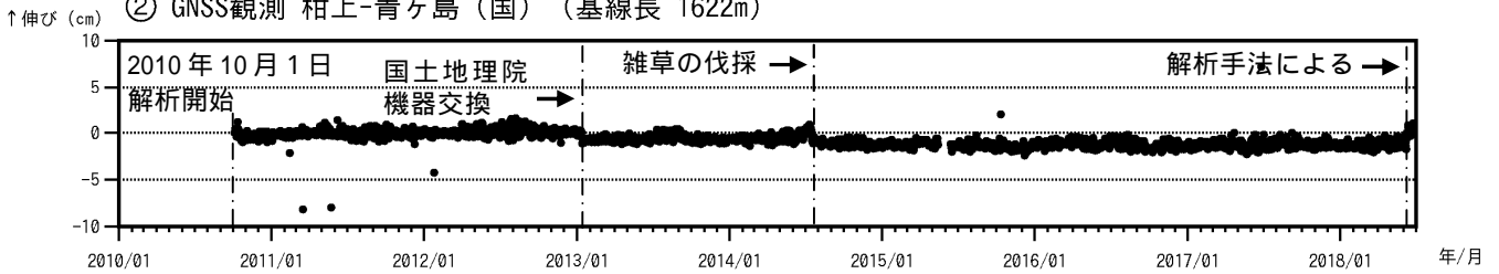
図2 青ヶ島 火山活動経過図(2010年8月9日~2018年6月30日)
