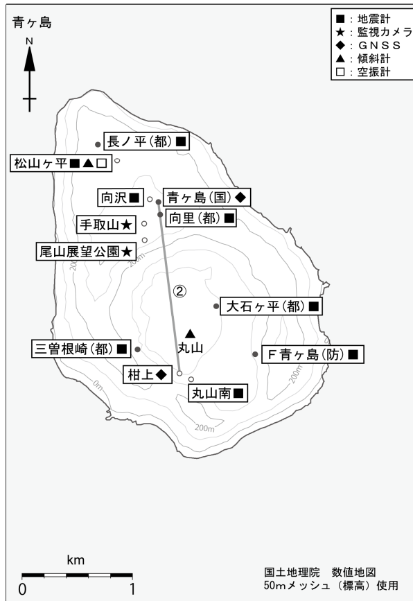
図3 青ヶ島 観測点配置図
