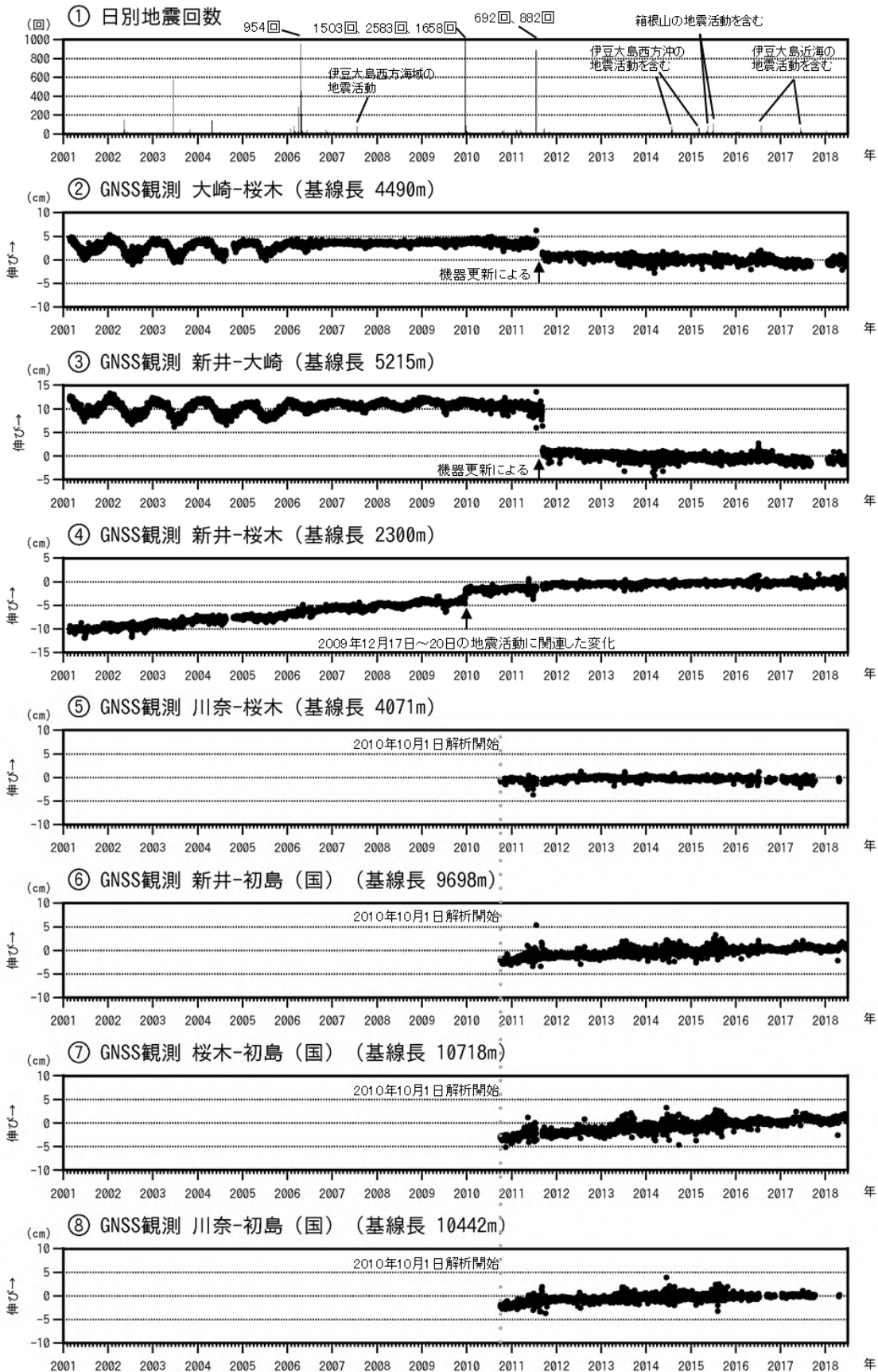
図3 伊豆東部火山群 火山活動経過図（2001年1月1日～2018年6月30日）
