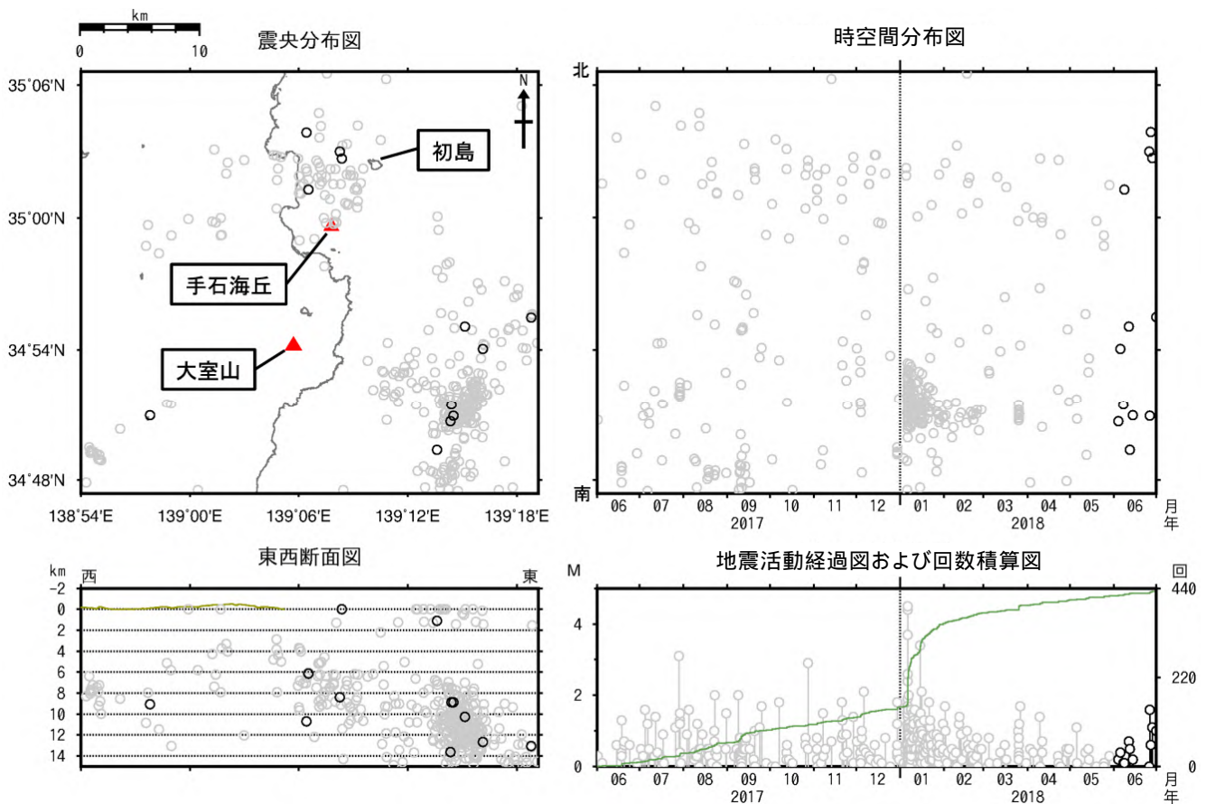
図2 伊豆東部火山群 広域地震観測網による震源分布図(2017年6月1日~2018年6月30日)
