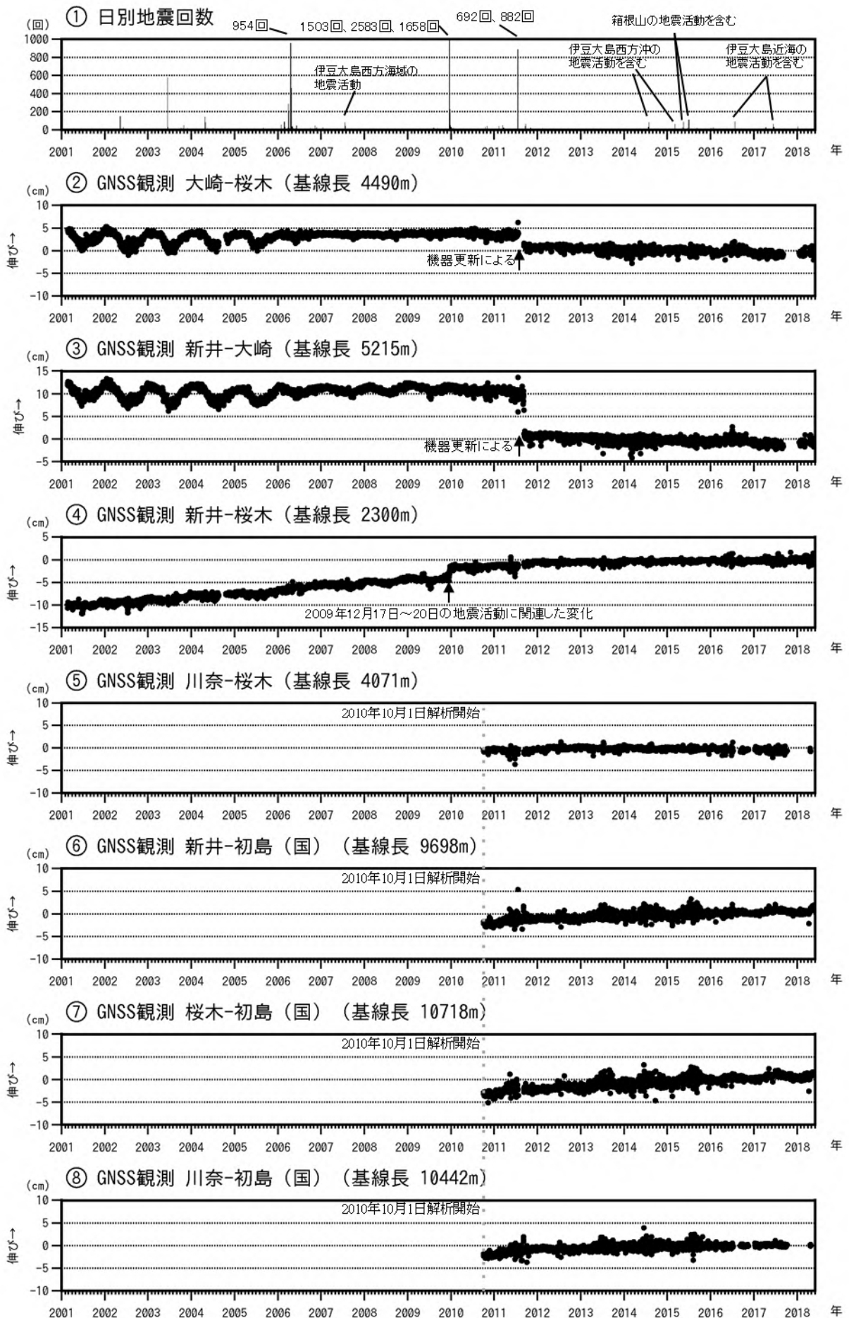
図3 伊豆東部火山群 火山活動経過図 (2001年1月1日~2018年5月31日)
