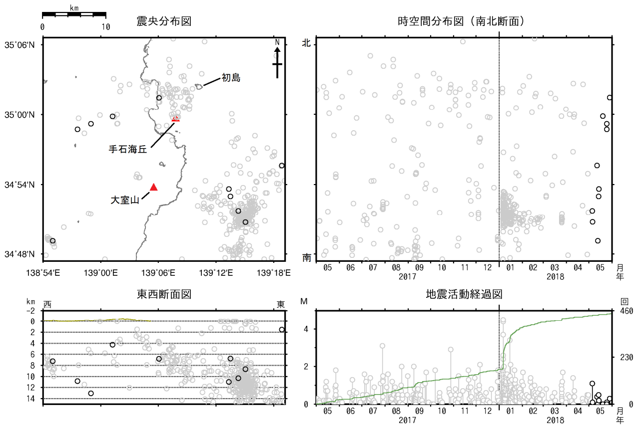
図2 伊豆東部火山群 広域地震観測網による震源分布図(2017年5月1日～2018年5月31日)
