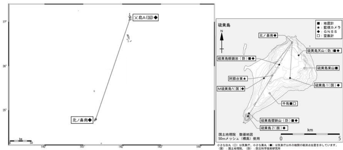
図7 硫黄島 観測点配置図
