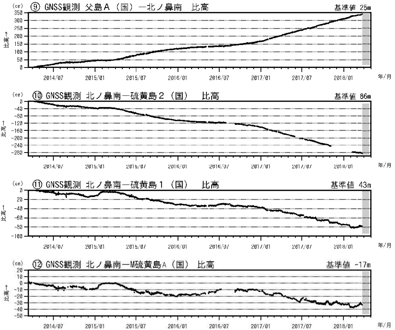
図6 硫黄島 GNSS 観測結果（2014年3月13日～2018年4月30日）
