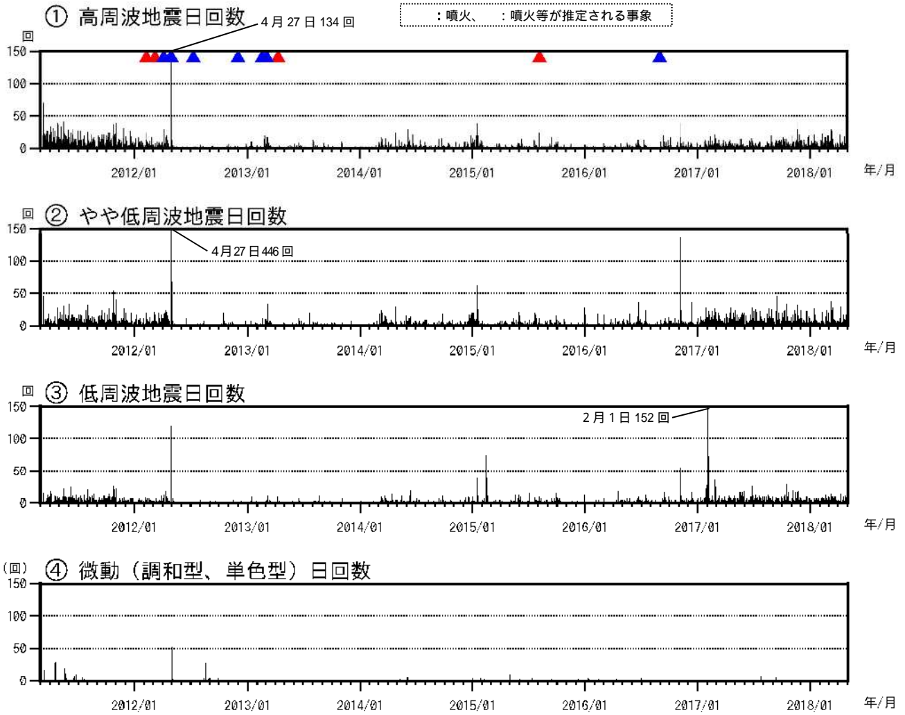
図4 硫黄島 火山活動経過図(2011年3月8日~2018年4月30日)
