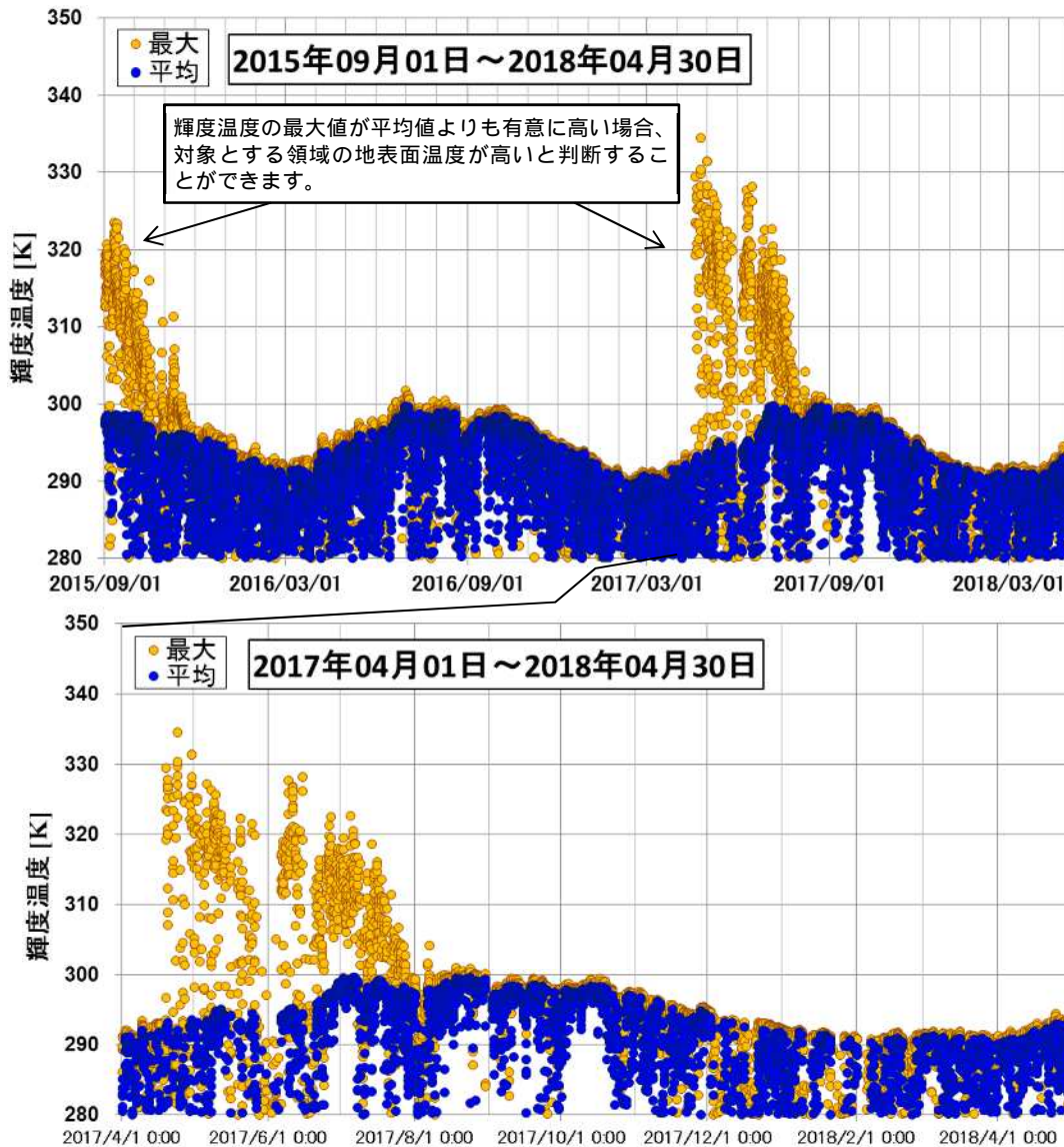
図 1 西之島 ひまわり 8 号の観測による西之島付近の輝度温度の変化
