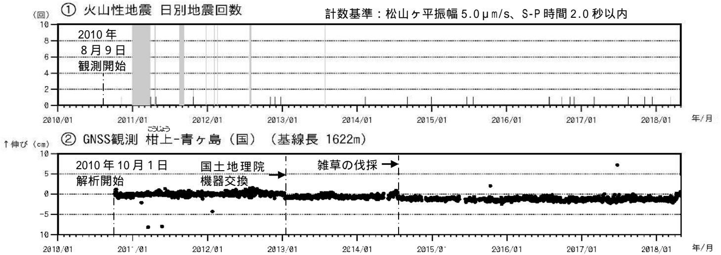
図2 青ヶ島 火山活動経過図(2010年8月9日~2018年4月30日)
