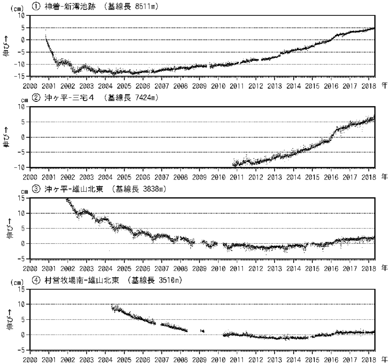
図7 三宅島 GNSS 連続観測結果(2000年10月26日~2018年4月30日)
