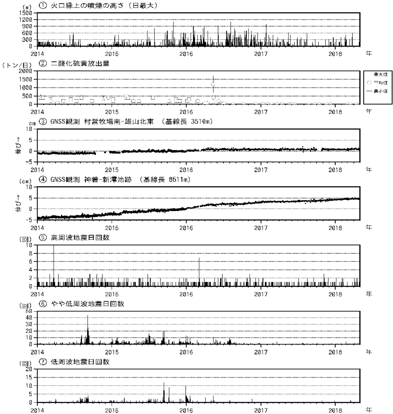
図6 三宅島 火山活動短期経過図（2014年1月1日～2018年4月30日）
