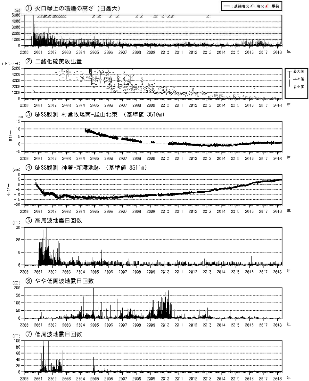
図5 三宅島 火山活動長期経過図（2000年1月1日～2018年4月30日）
