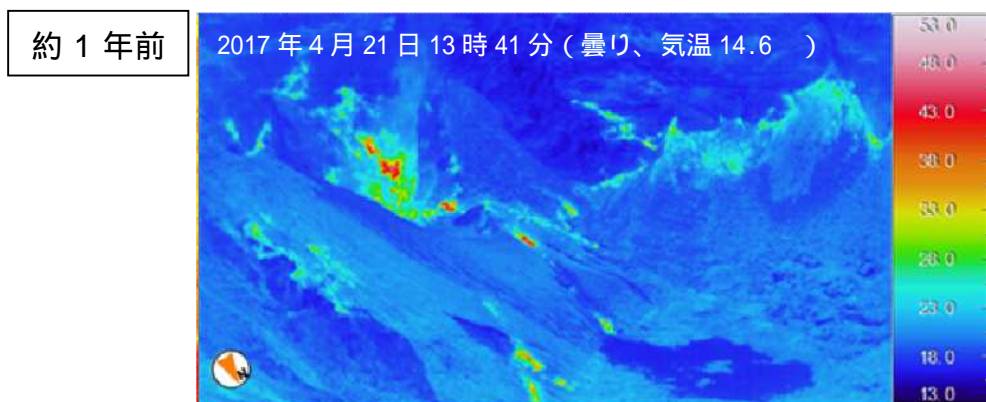
図 4 三宅島 赤外熱映像装置による山頂火口内の地表面温度分布 ・ 3 日に実施した現地調査では、3 月や昨年と同様に主火孔内及びその周辺で引き続き高温領域が認められました。高温領域の分布に特段の変化は認められません。
