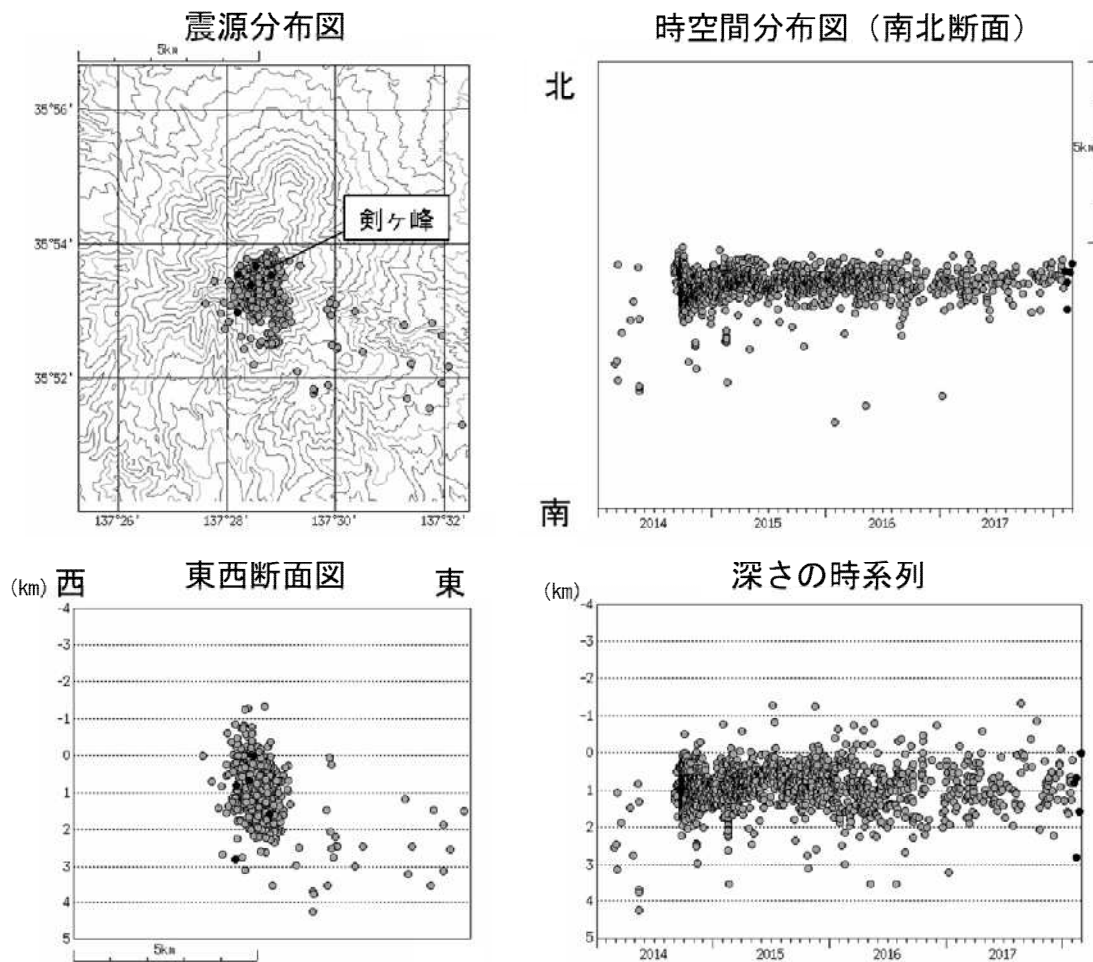
図2 御嶽山 震源分布図(2014年1月1日~2018年2月28日)
