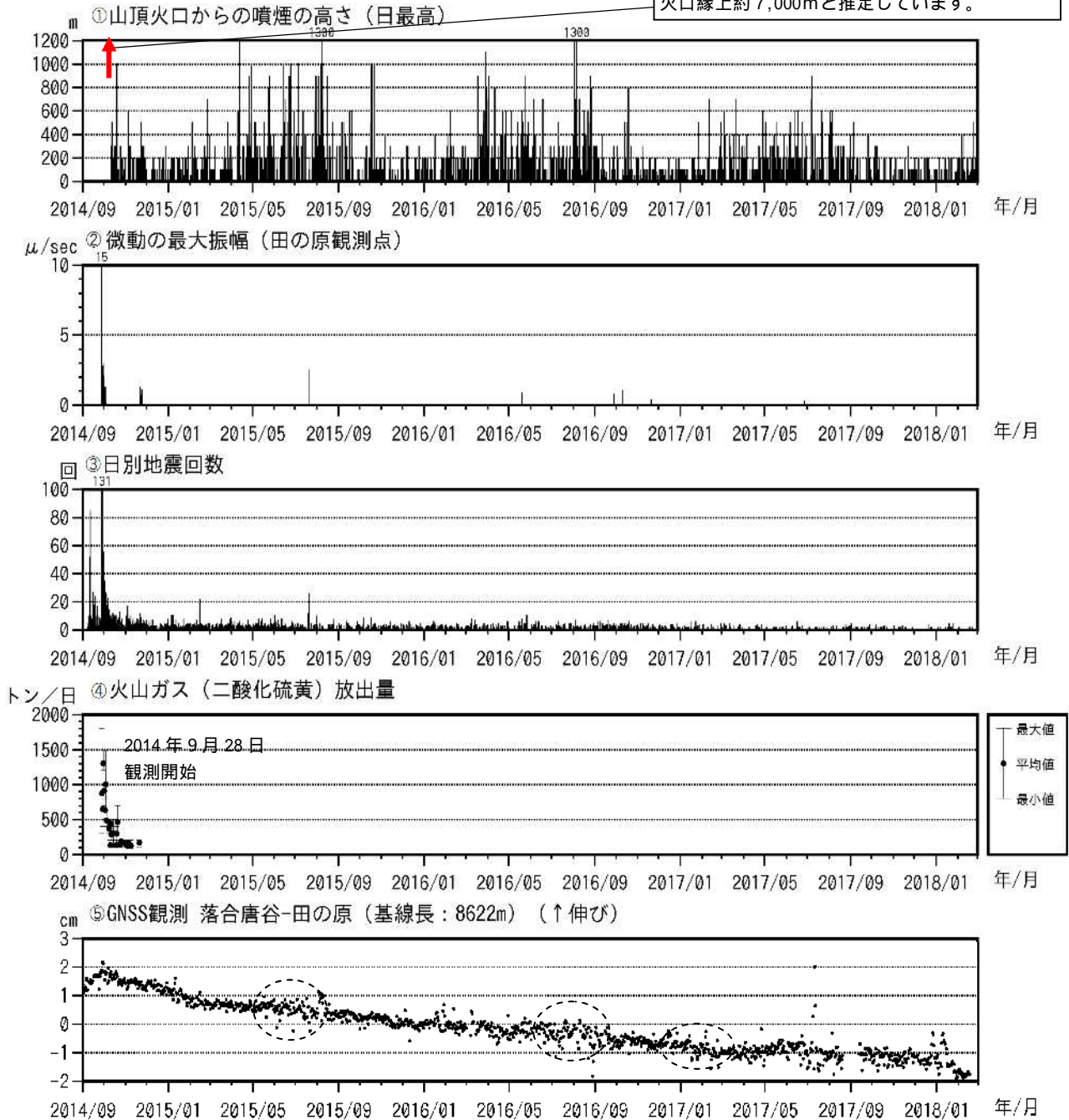
図3 御嶽山 最近の火山活動経過図(2014年9月1日~2018年2月28日)
