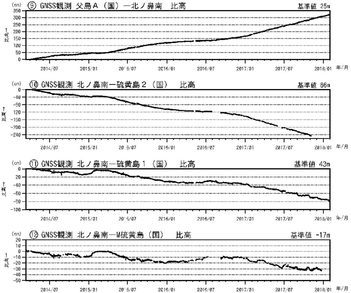
図6 硫黄島 GNSS観測結果(2014年3月13日~2018年1月31日) (国): 国土地理院、比高: 左の観測点に対する右の観測点の高度の差、空白部分は欠測 図7の ~ に対応。
