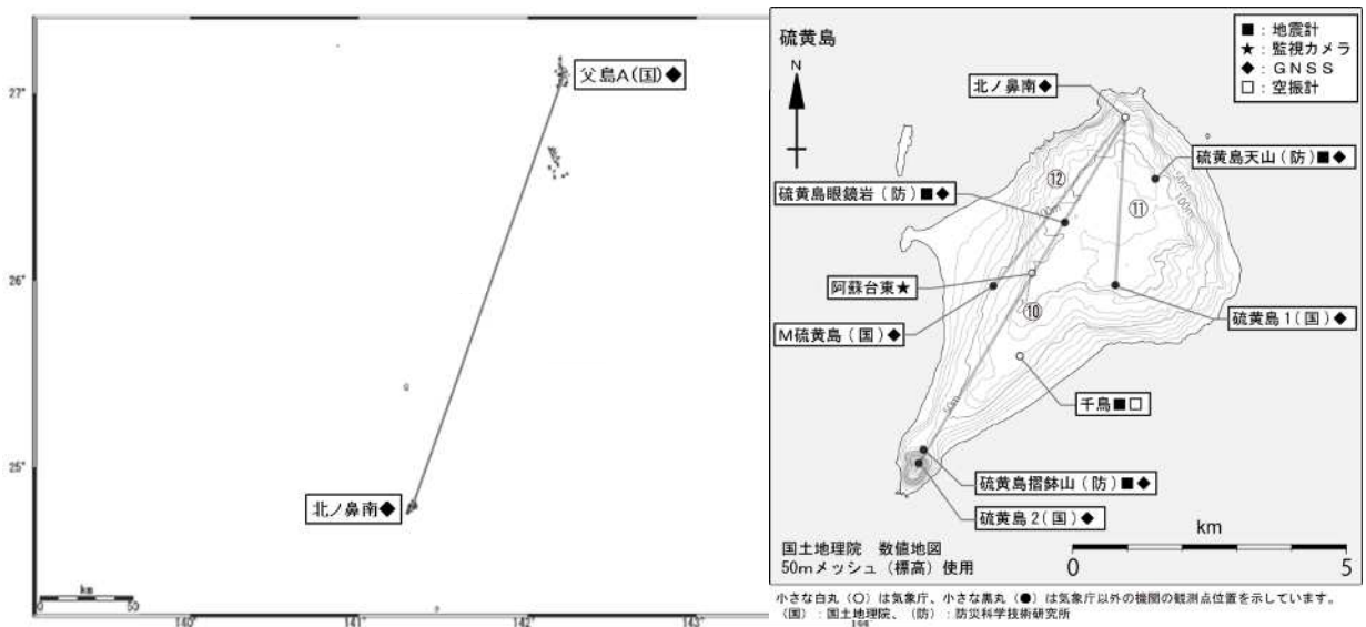
図7 硫黄島 観測点配置図 小さな白丸(O)は気象庁、小さな黒丸(●)は気象庁以外の機関の観測点位置を示しています。 図中の灰色線 ~ は図6の基線 ~ に対応、(国): 国土地理院。
