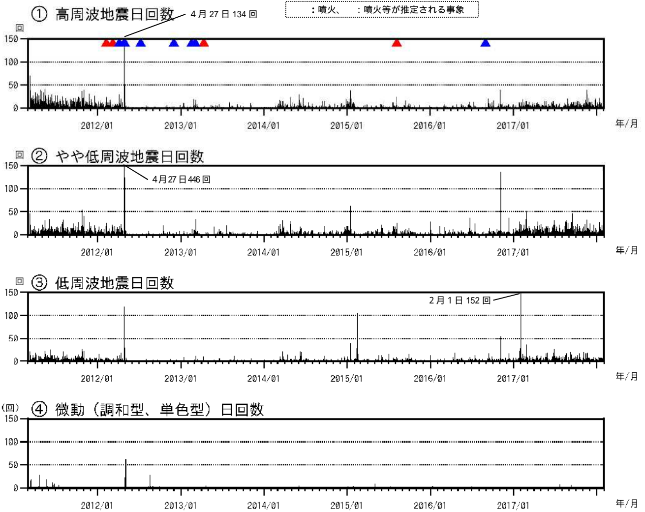
図4 硫黄島 火山活動経過図(2011年3月8日~2018年1月31日)
