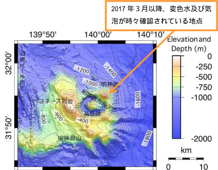
図 2 ベヨネース列岩付近の海底地形図と
