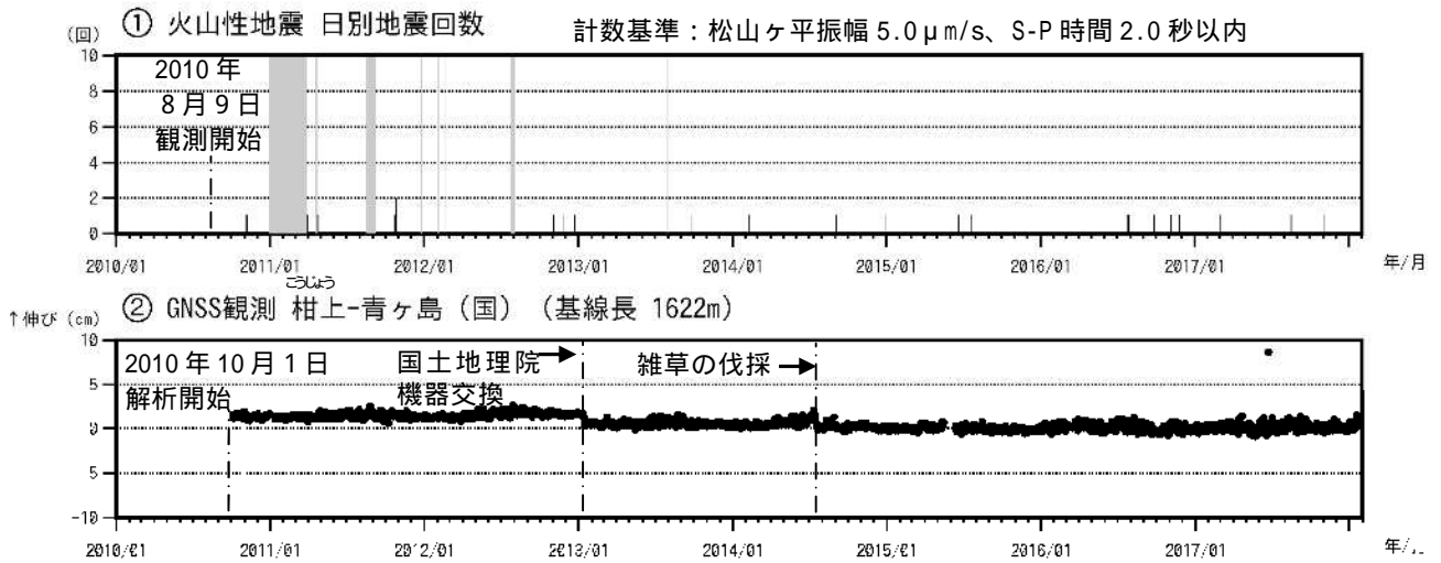
図2 青ヶ島 火山活動経過図(2010年8月9日~2018年1月31日)
