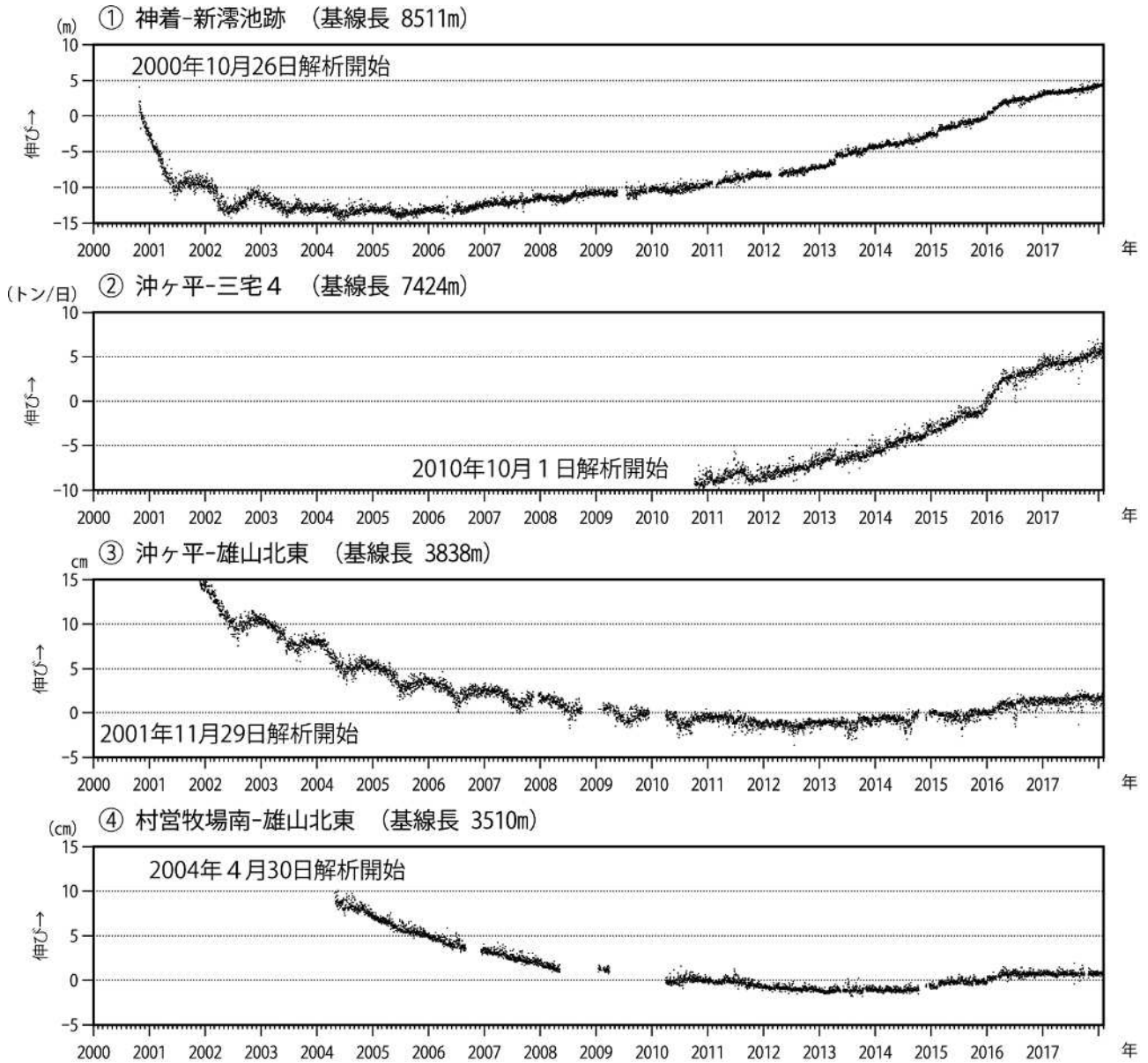
図7 三宅島 GNSS 連続観測結果 (2000年10月26日~2018年1月31日)
