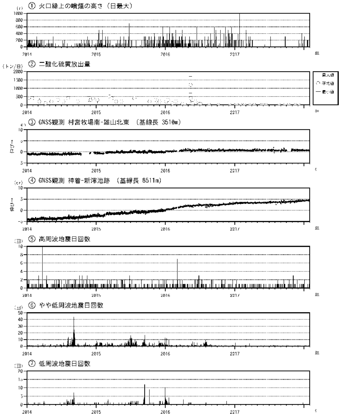
図6 三宅島 火山活動短期経過図(2014年1月1日~2018年1月31日)
