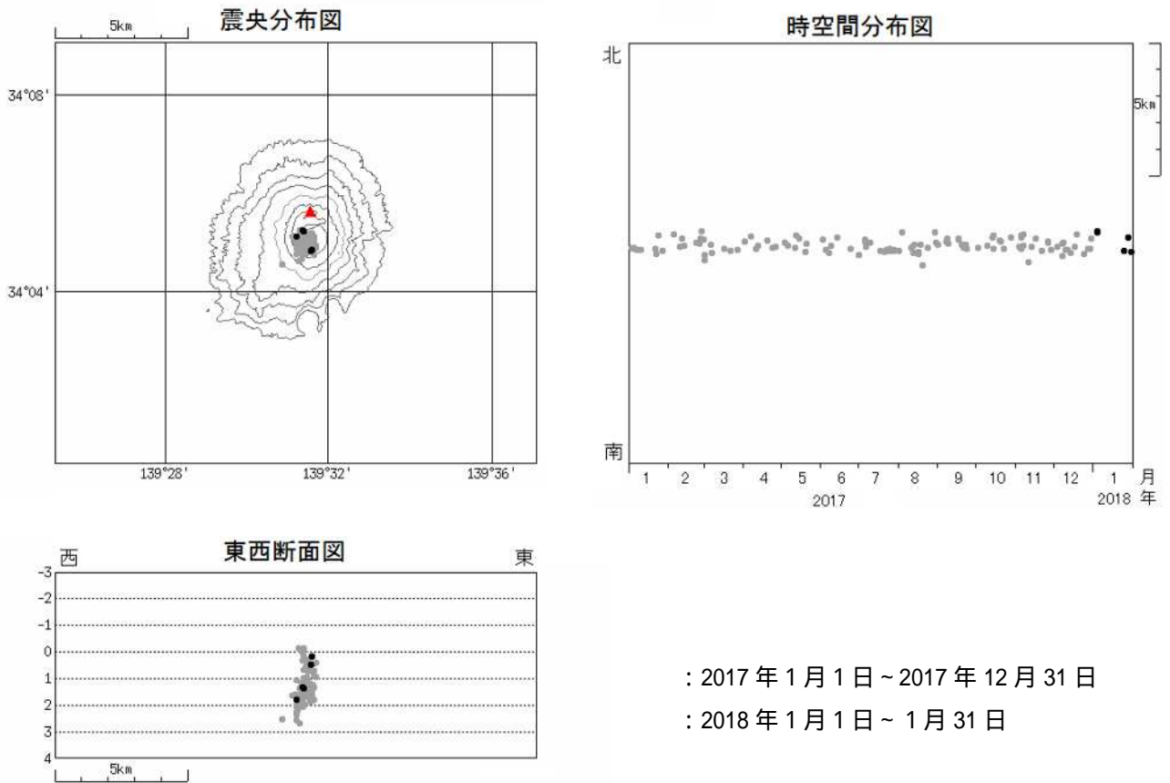
図8 三宅島 震源分布図(2017年1月1日~2018年1月31日)
