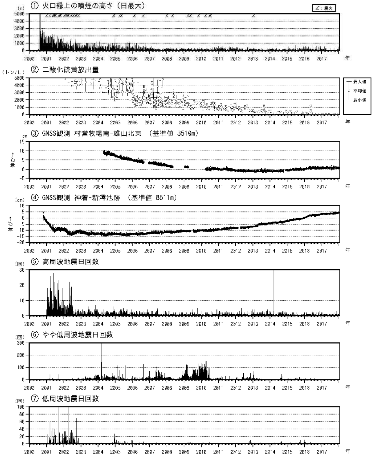
図5 三宅島 火山活動長期経過図(2000年1月1日~2018年1月31日)
