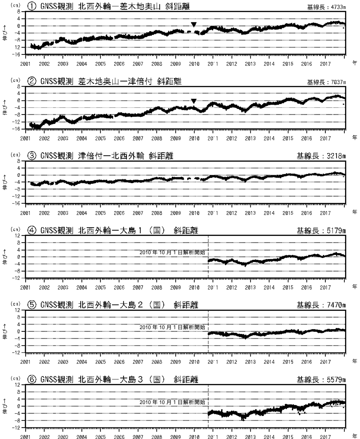
図3 伊豆大島 GNSS連続観測による基線長変化(2001年1月~2018年1月31日)
