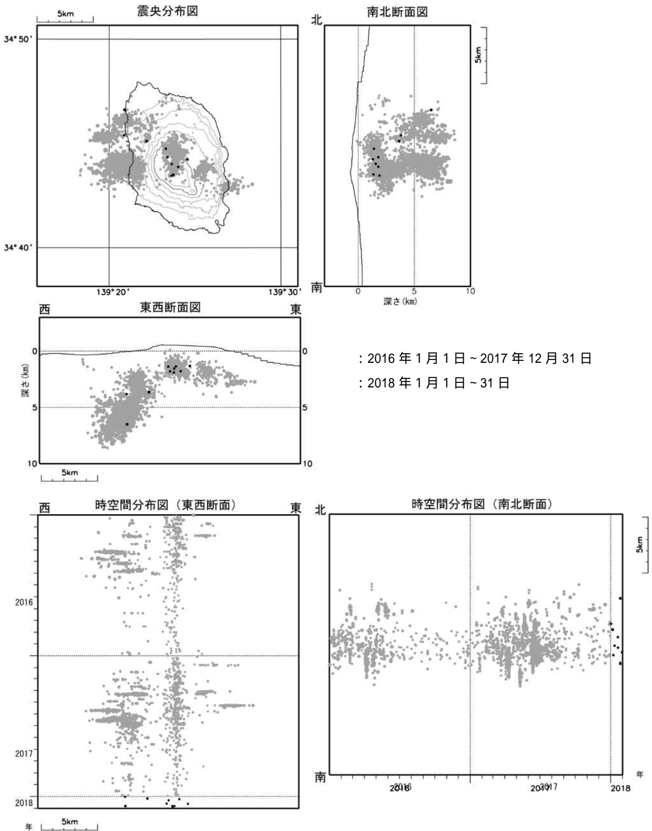
図 4 伊豆大島 震源分布図（2016 年 1 月 1 日 ~ 2018 年 1 月 31 日）
