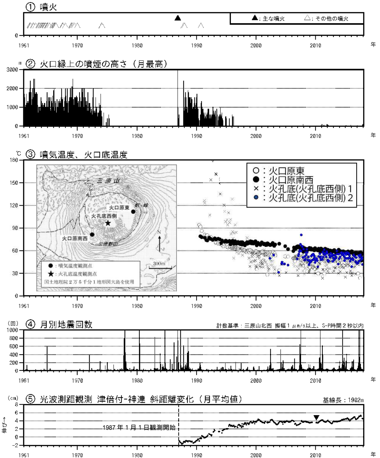
図1 伊豆大島 長期間の火山活動経過図(1961年1月~2018年1月31日)
