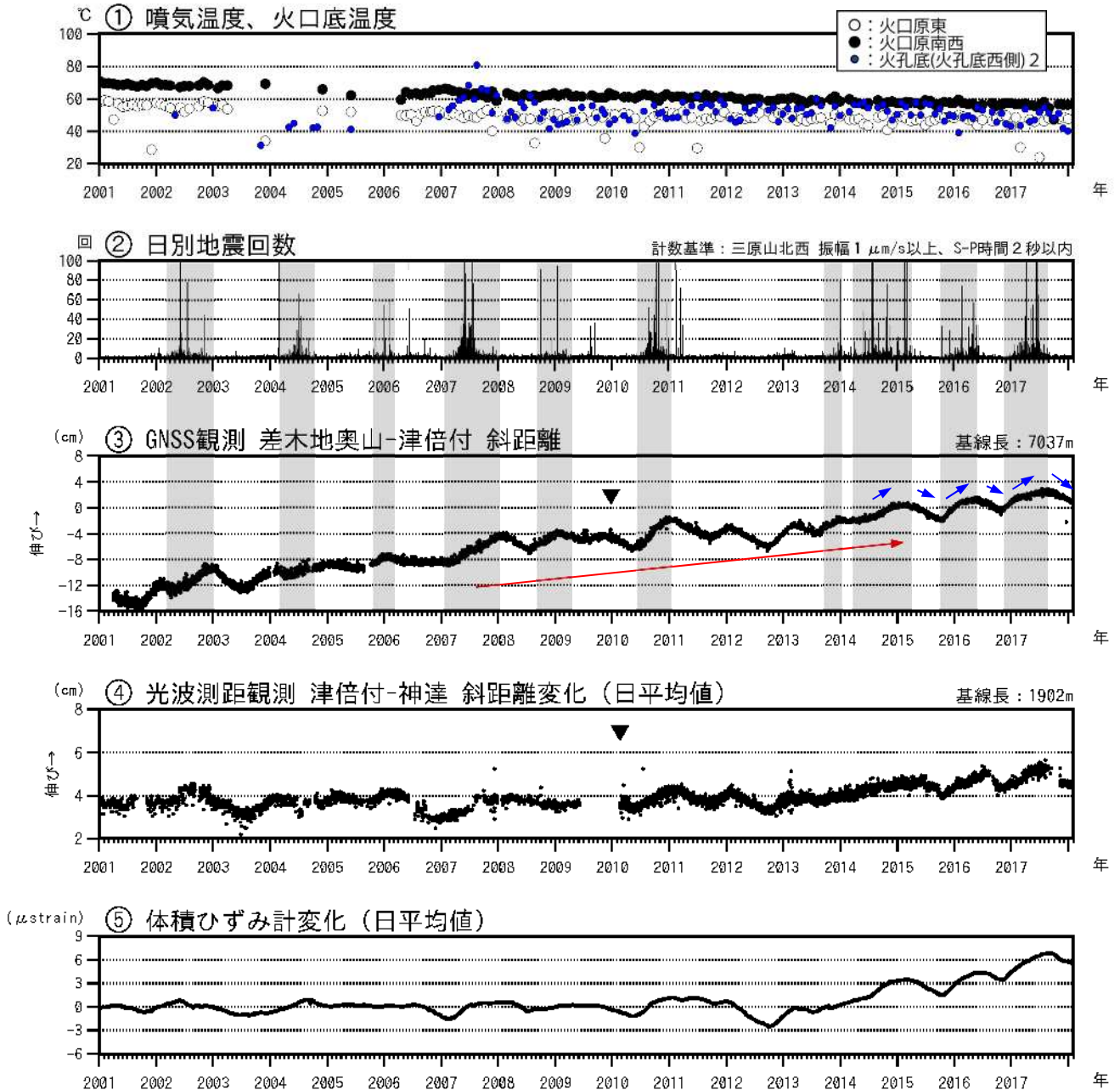
図2 伊豆大島 最近の火山活動経過図(2001年1月~2018年1月31日)
