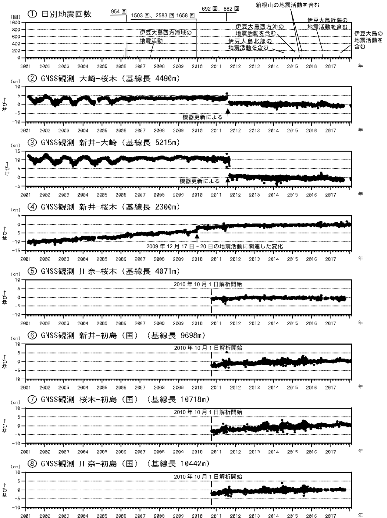
図3 伊豆東部火山群 火山活動経過図(2001年1月1日~2018年1月31日)
