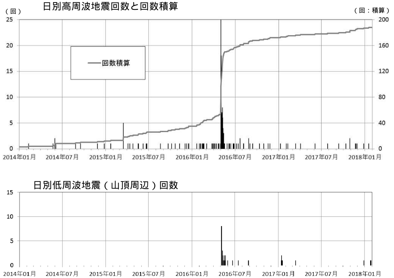
図6 新潟焼山 日別地震回数(2014年1月1日~2018年1月31日)
