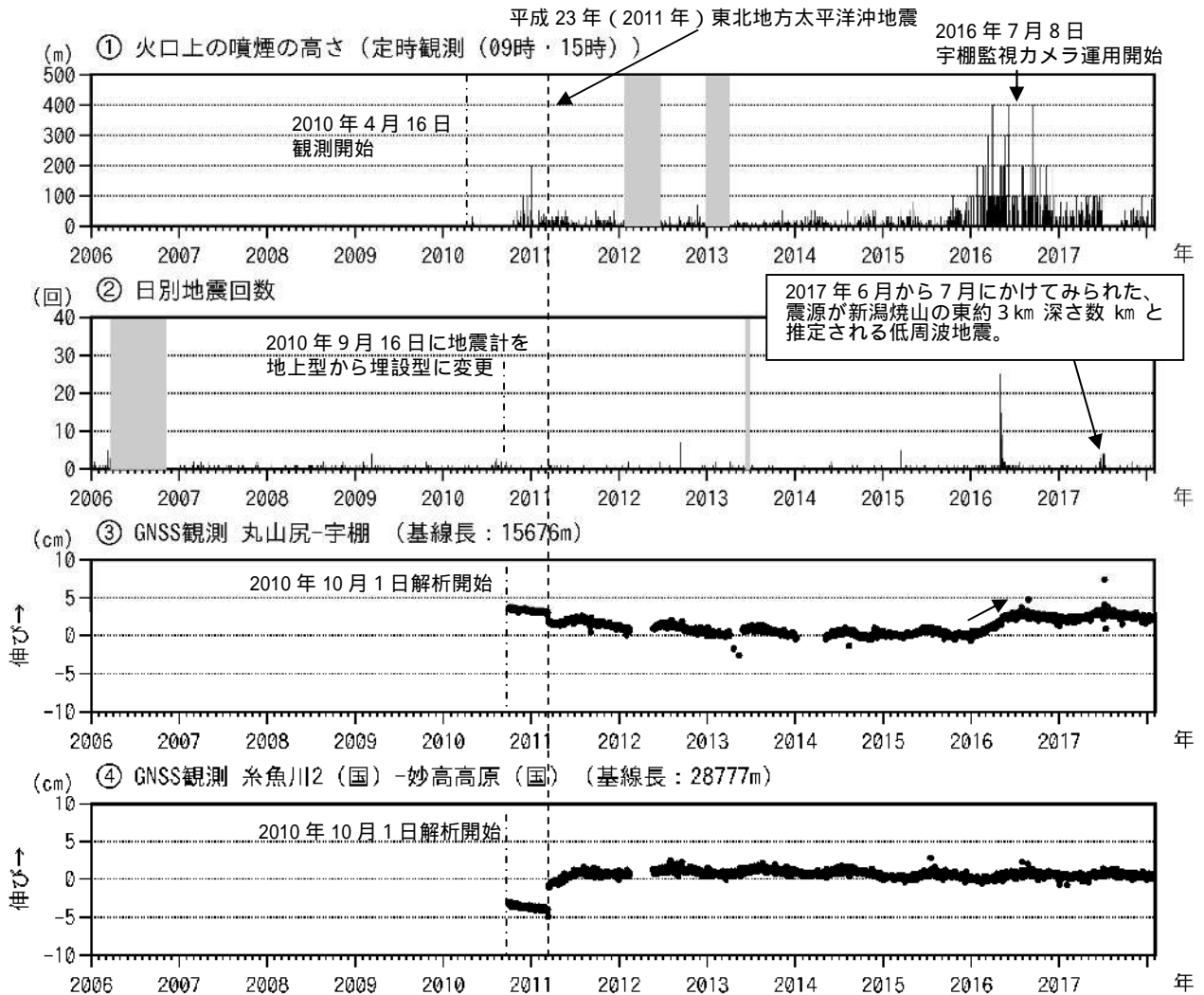
図3 新潟焼山 火山活動経過図(2006年1月1日~2018年1月31日)
