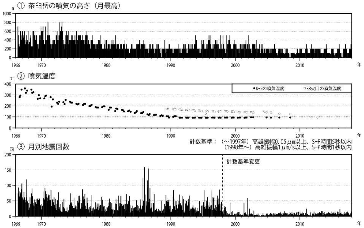
図2 那須岳 火山活動経過図(1966年1月～2018年1月)
