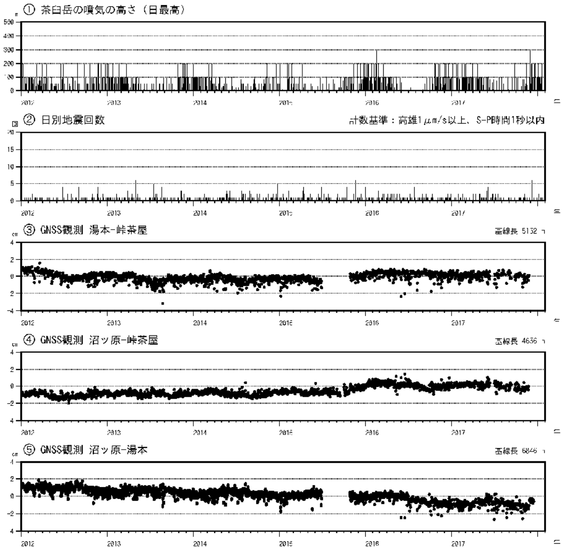
図3 那須岳 火山活動経過図(2012年1月1日~2018年1月31日)
