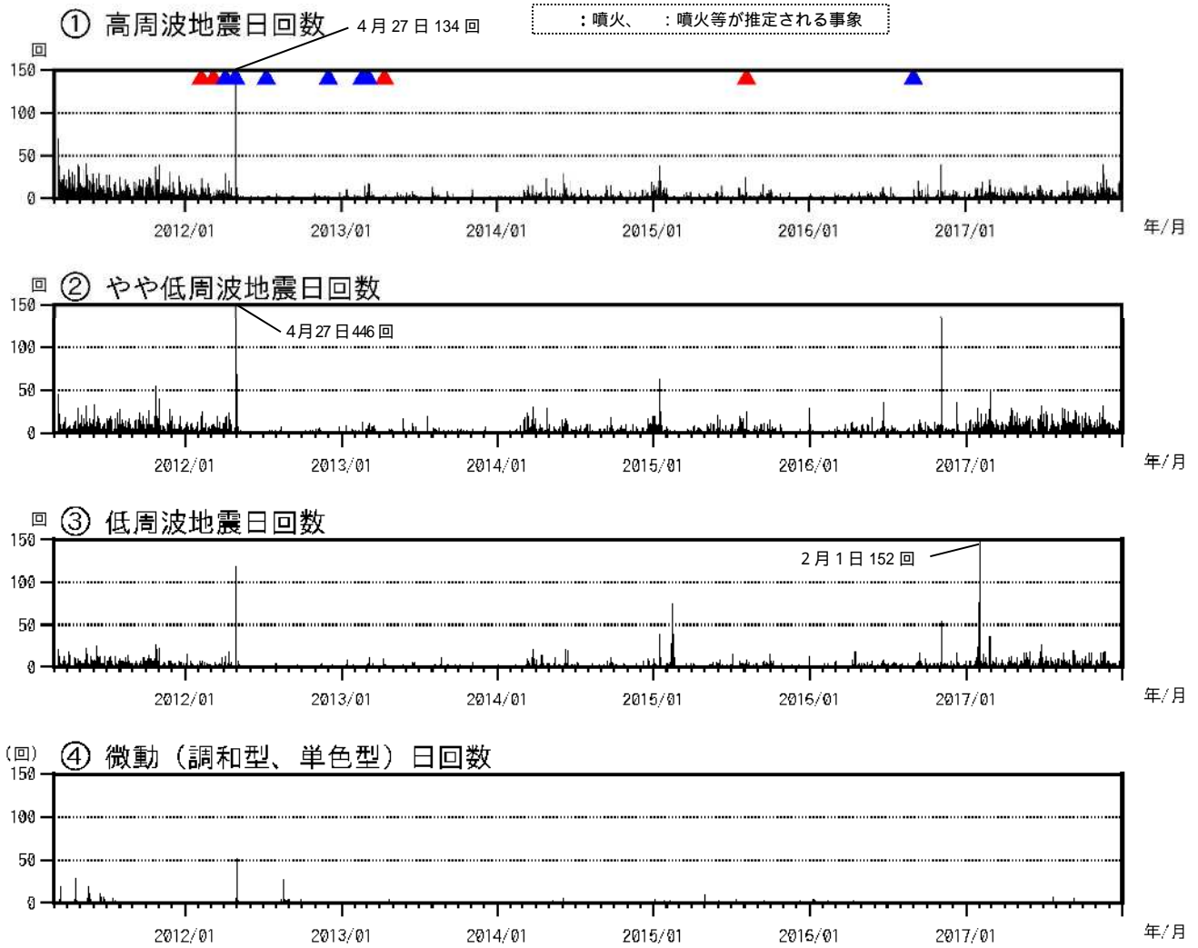
図4 硫黄島 火山活動経過図（2011年3月8日～2017年12月31日）
