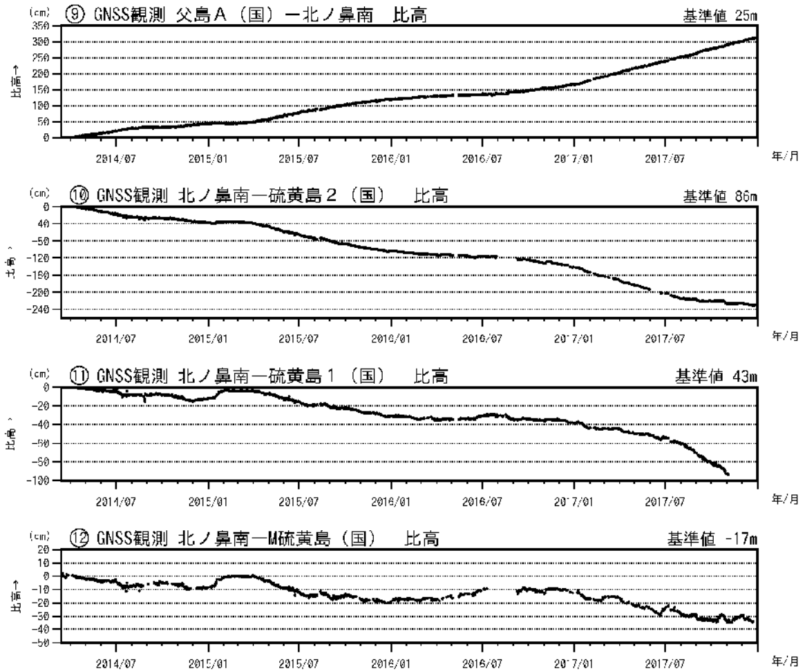
図6 硫黄島 GNSS 観測結果（2014年3月13日～2017年12月31日）
