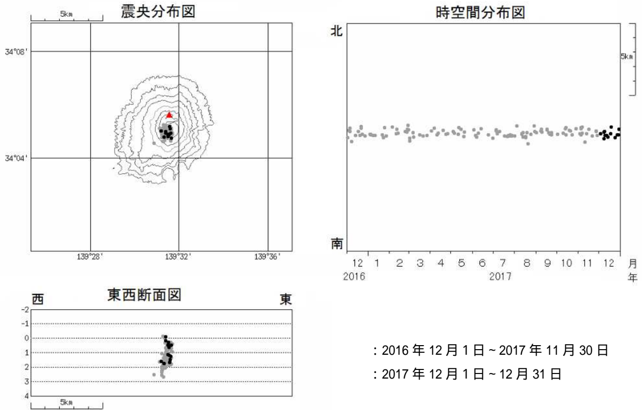
図8 三宅島 震源分布図(2016年12月1日~2017年12月31日) ・震源は山頂火口直下に分布しており、これまでと比べて特段の変化は認められません。
