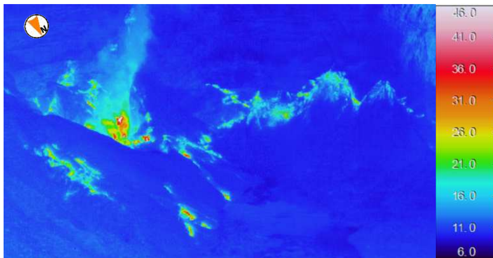
図 4 三宅島 赤外熱映像装置による山頂火口内の地表面温度分布
