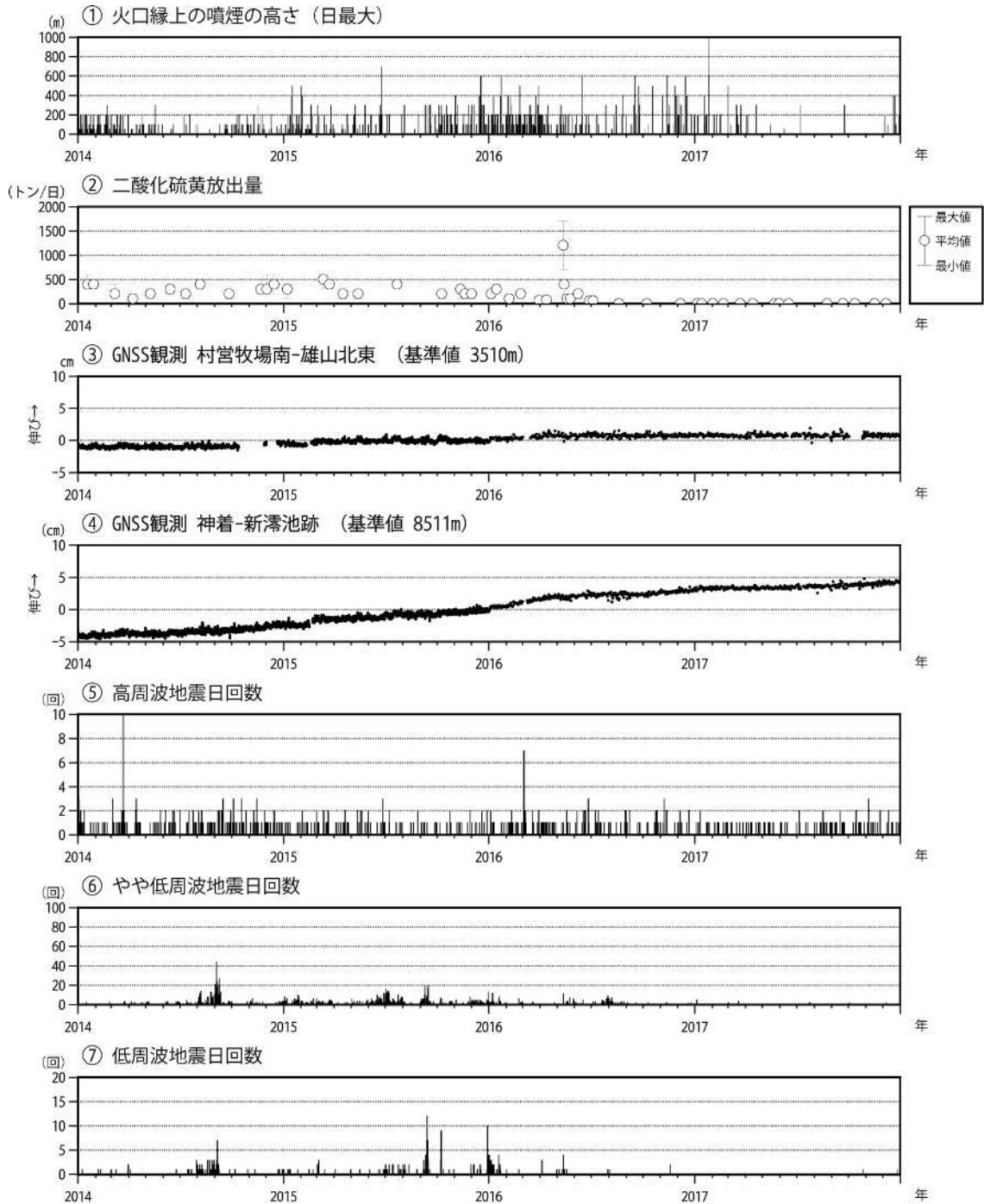
図6 三宅島 火山活動短期経過図（2014年1月1日～2017年12月31日）
