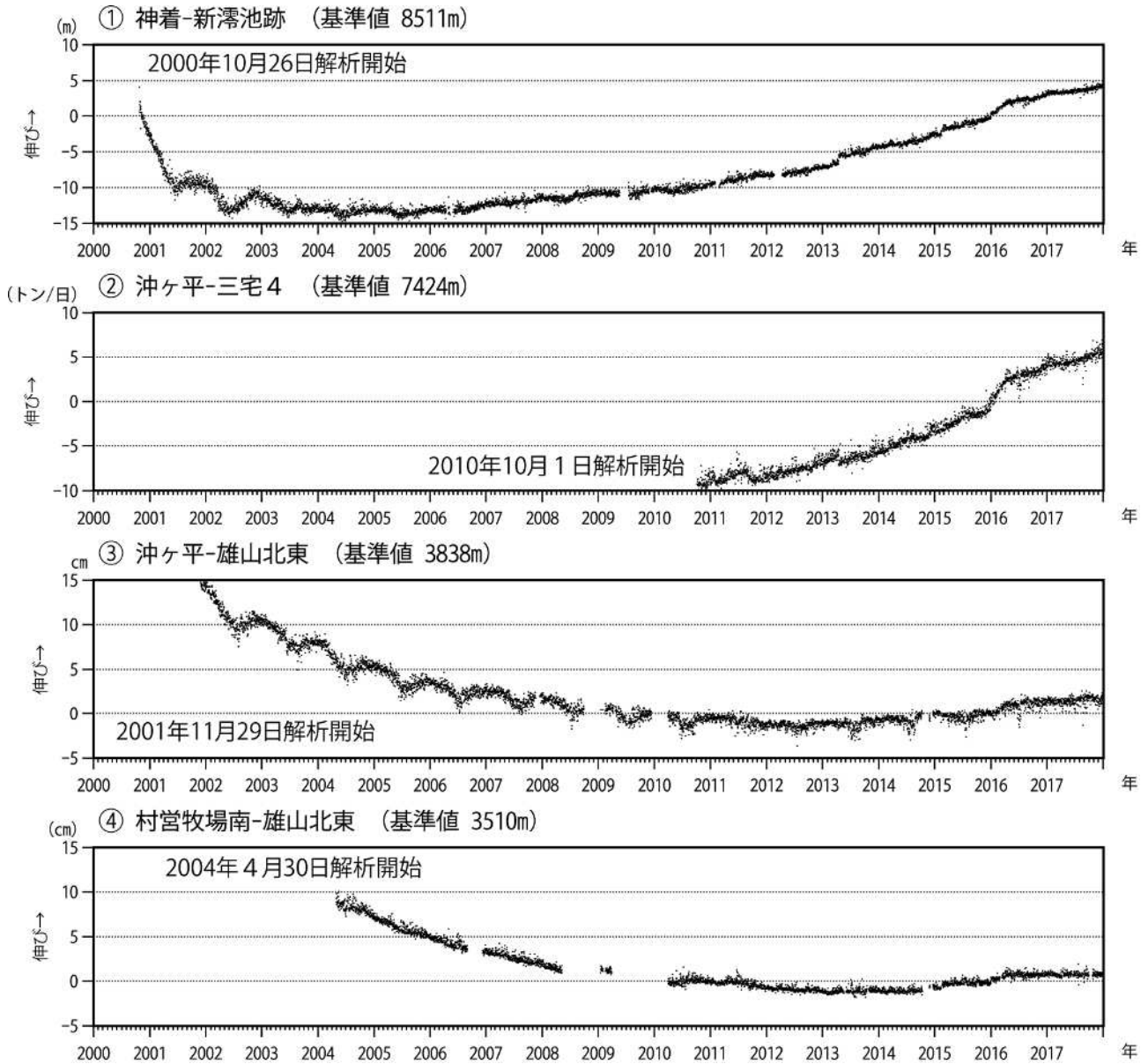
図7 三宅島 GNSS 連続観測結果（2000年10月26日～2017年12月31日）
