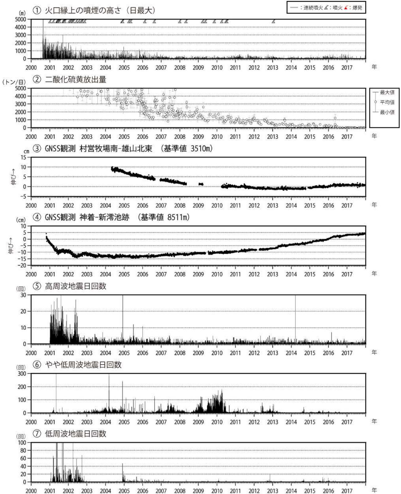
図5 三宅島 火山活動長期経過図（2000年1月1日～2017年12月31日）
