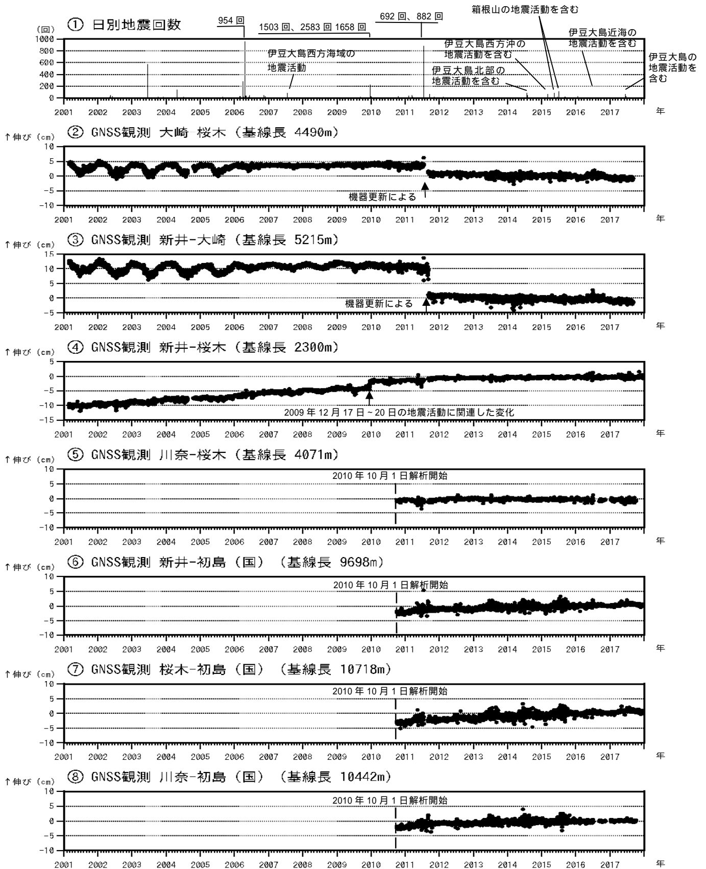
図3 伊豆東部火山群 火山活動経過図(2001年1月1日~2017年12月31日)
