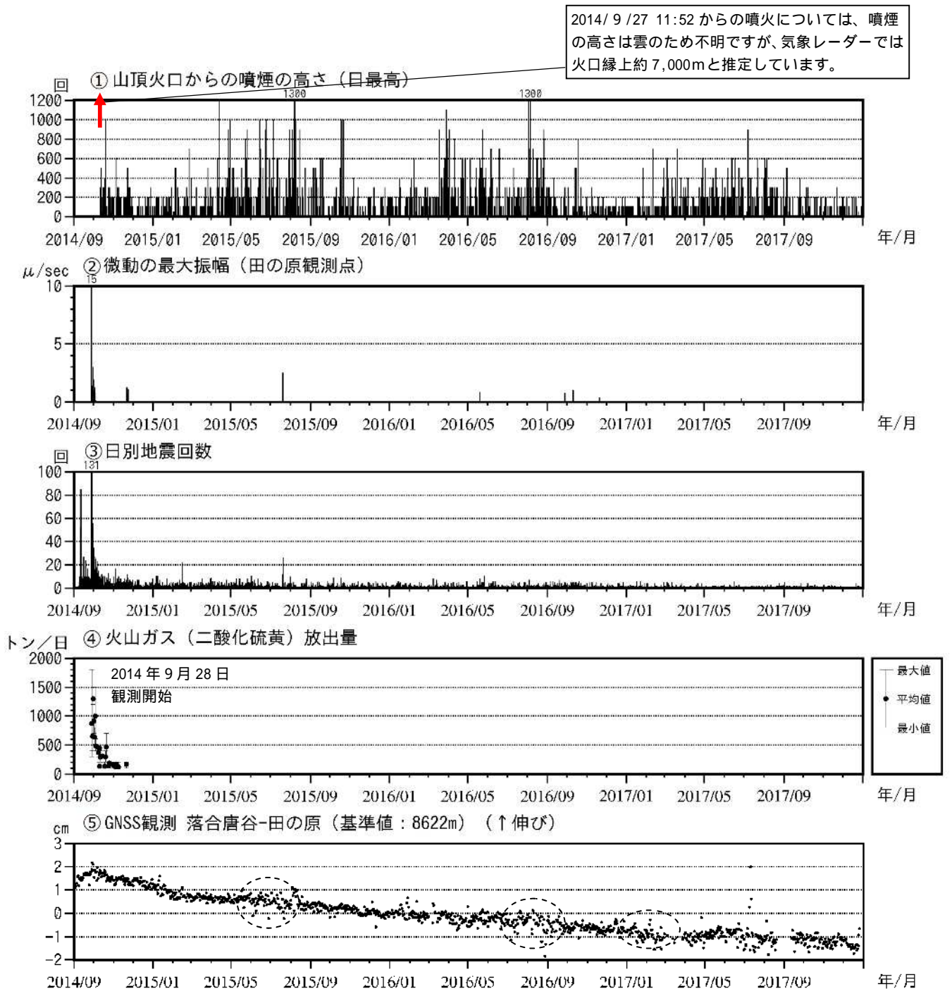
図3 御嶽山 最近の火山活動経過図（2014年9月1日～2017年12月31日）
