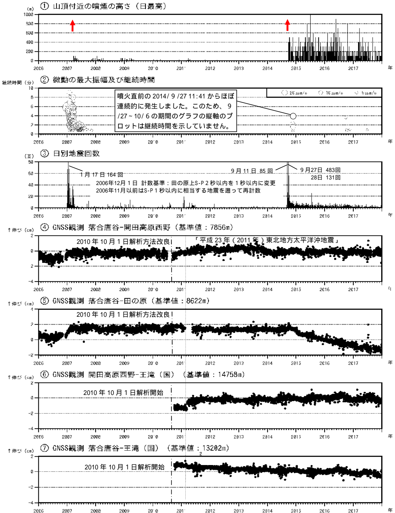
図4 御嶽山 長期間の火山活動経過図（2006年1月1日～2017年12月31日）
