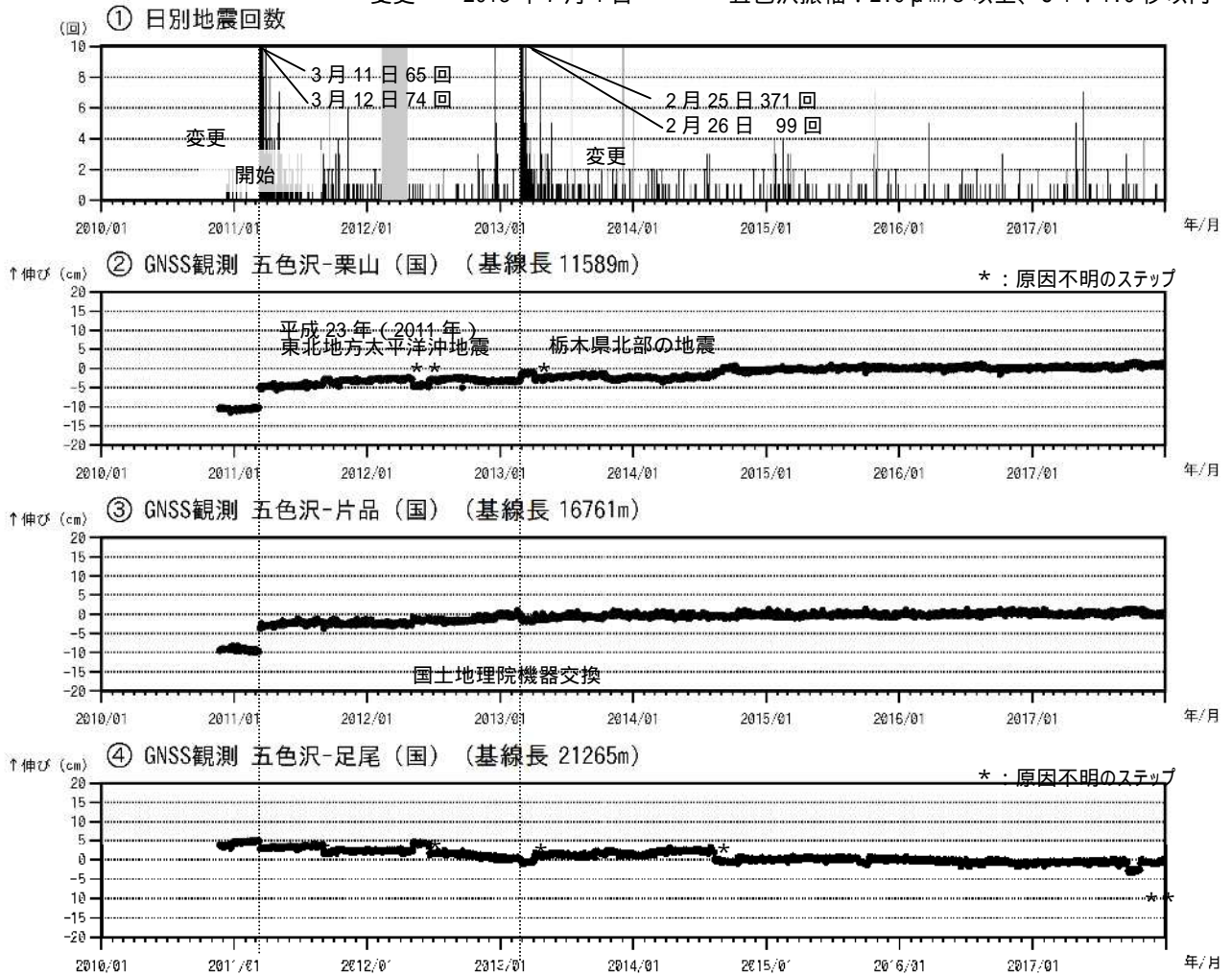
図2 日光白根山 火山活動経過図(2010年11月20日～2017年12月31日)
