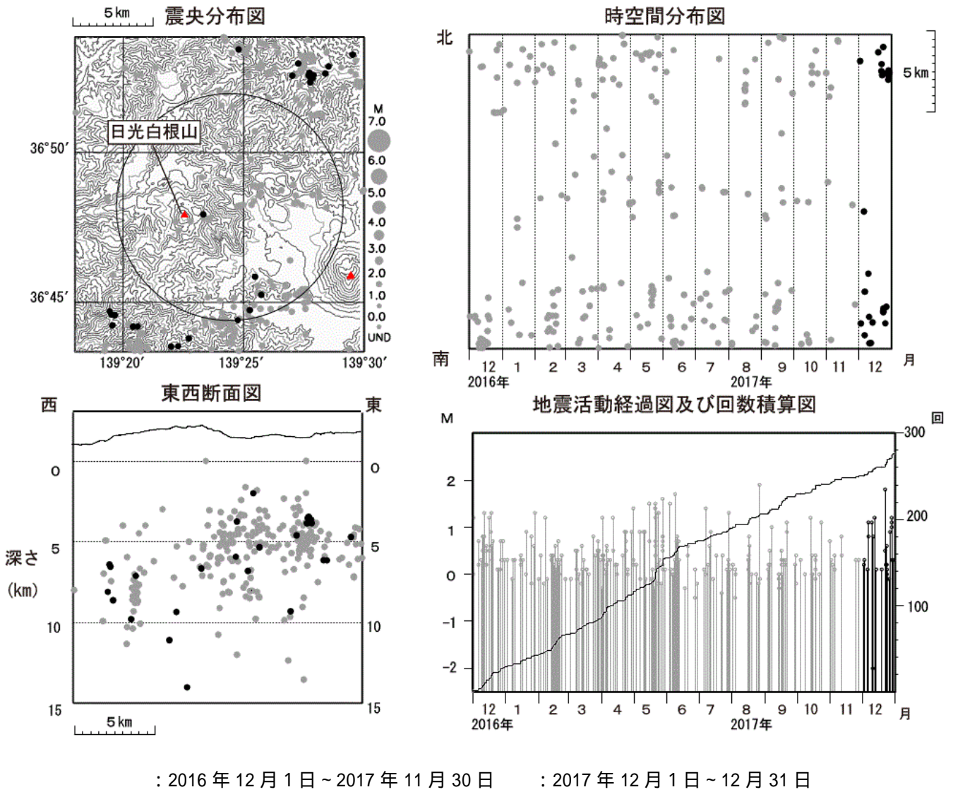
図 3 日光白根山 広域地震観測網による山体・周辺の地震活動 (2016 年 12 月 1 日 ~ 2017 年 12 月 31 日)
