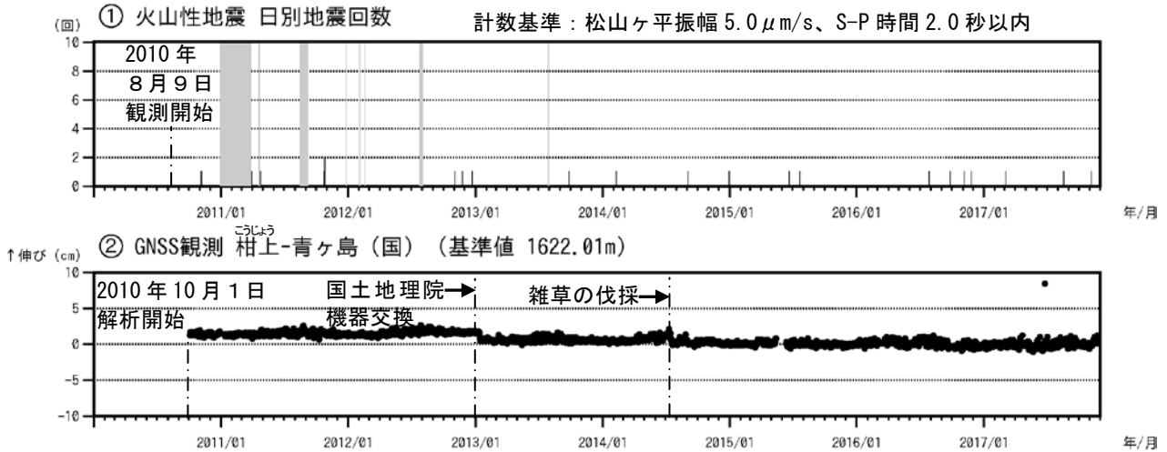
図2 青ヶ島 火山活動経過図 (2010年8月9日~2017年11月30日)
