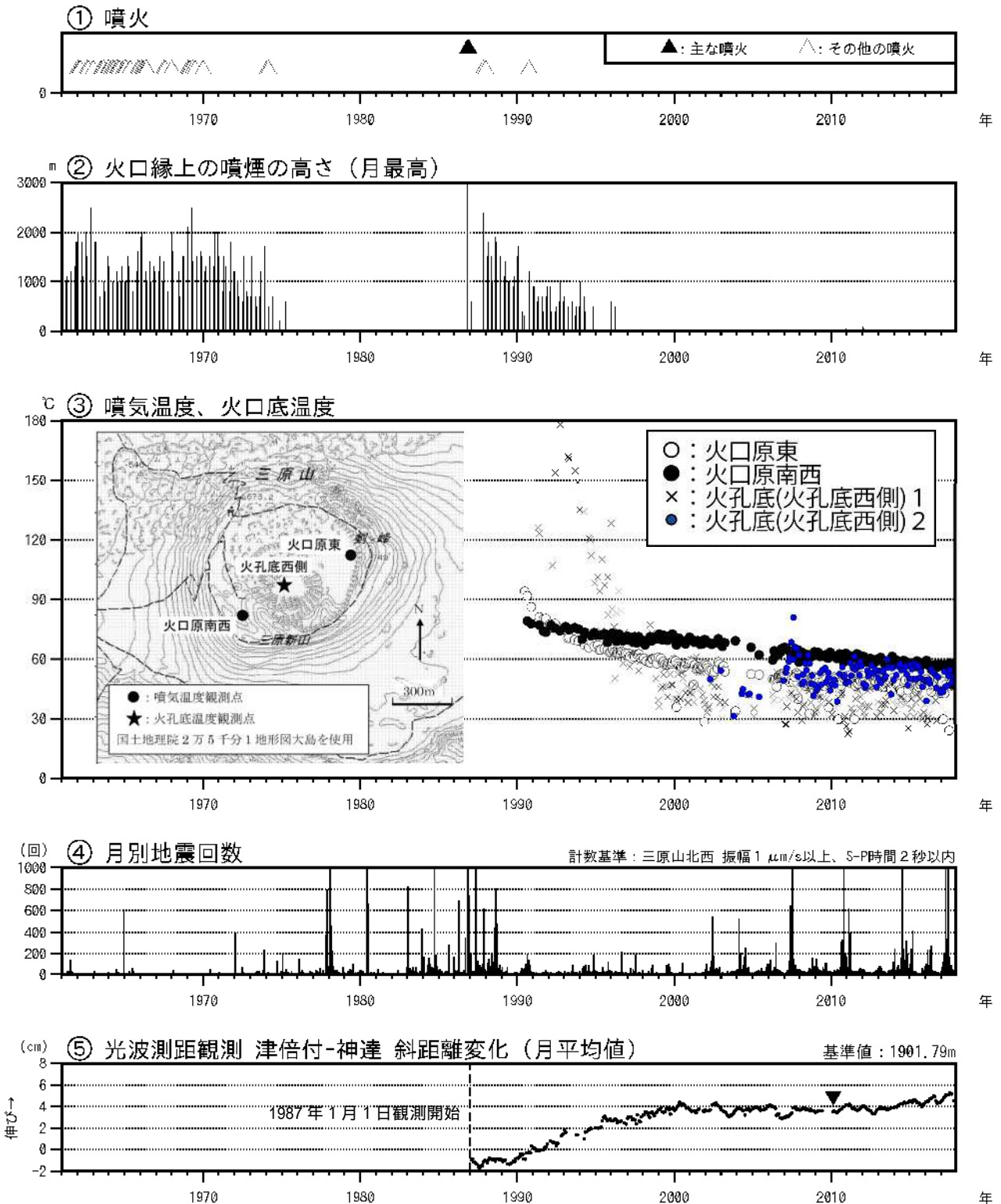
図 1 伊豆大島 長期間の火山活動経過図（1961 年 1 月～2017 年 11 月 30 日）
