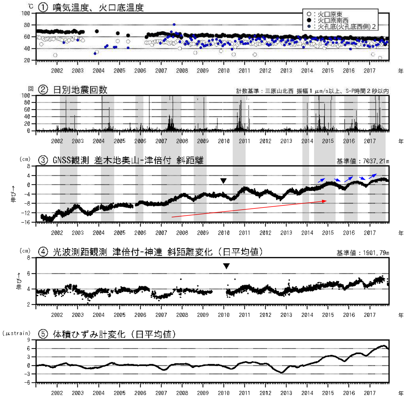
図 2 伊豆大島 最近の火山活動経過図（2001 年 1 月～2017 年 11 月 30 日）
