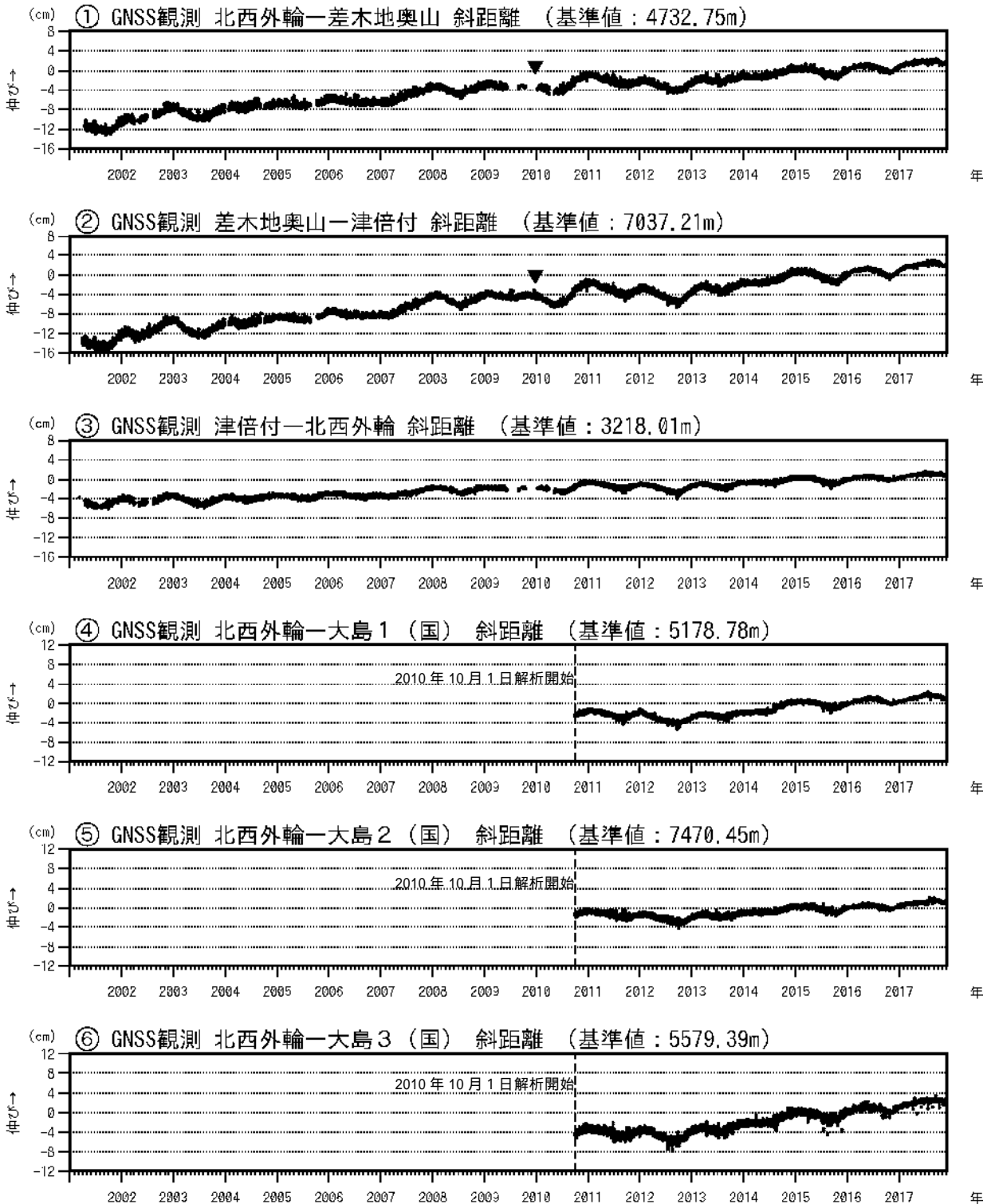
図3 伊豆大島 GNSS連続観測による基線長変化(2001年1月~2017年11月30日)
