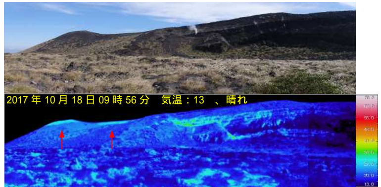
図 10 伊豆大島 剣ガ峰付近に確認された熱異常域の状況 ・前回（10月18日）確認された熱異常域は、今回は認められませんでした（図中赤矢印）。
