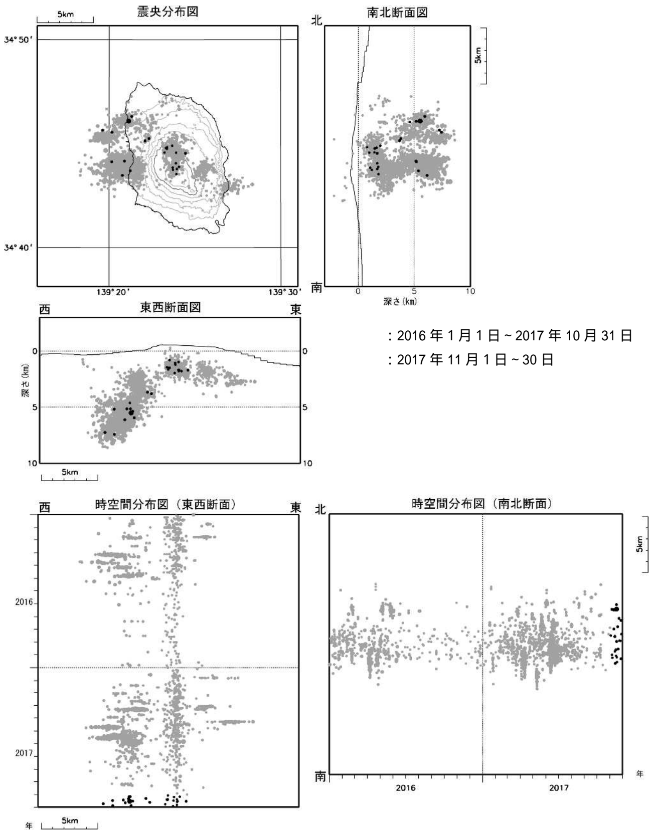
図4 伊豆大島 震源分布図（2016年1月1日～2017年11月30日） ・震源は、三原山周辺の浅いところと西方沖に分布しています。
