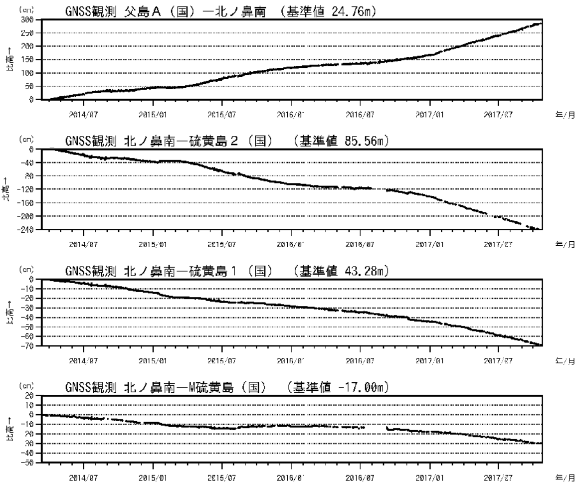
図6 硫黄島 GNSS 観測結果(2014年3月13日~2017年10月31日) (国): 国土地理院 ・基線 ~ は図7の ~ に対応します。いずれの図も、左の観測点に対する右の観測点の比高(高度の差)の変化を表しています。グラフの空白部分は欠測を示します。
