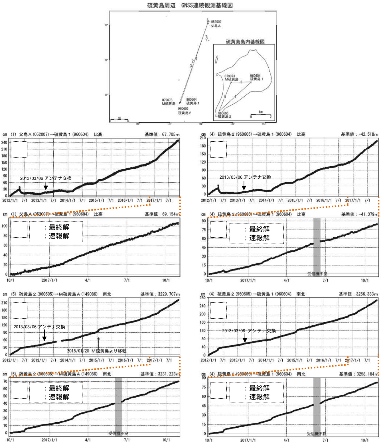
図5 硫黄島 国土地理院による地殻変動観測結果 2) ( 2012年1月1日~2017年10月29日、 2016年10月1日~2017年10月29日 ) のグラフ: 父島に対する硫黄島1の比高の変化 のグラフ: 硫黄島2(島南西部の摺鉢山付近)に対する硫黄島1(島北部の元山地域)の比高の変化 のグラフ: 硫黄島2に対するM硫黄島(島西部の阿蘇台陥没孔付近)の南北の変化 のグラフ: 硫黄島2に対する硫黄島1の南北の変化
