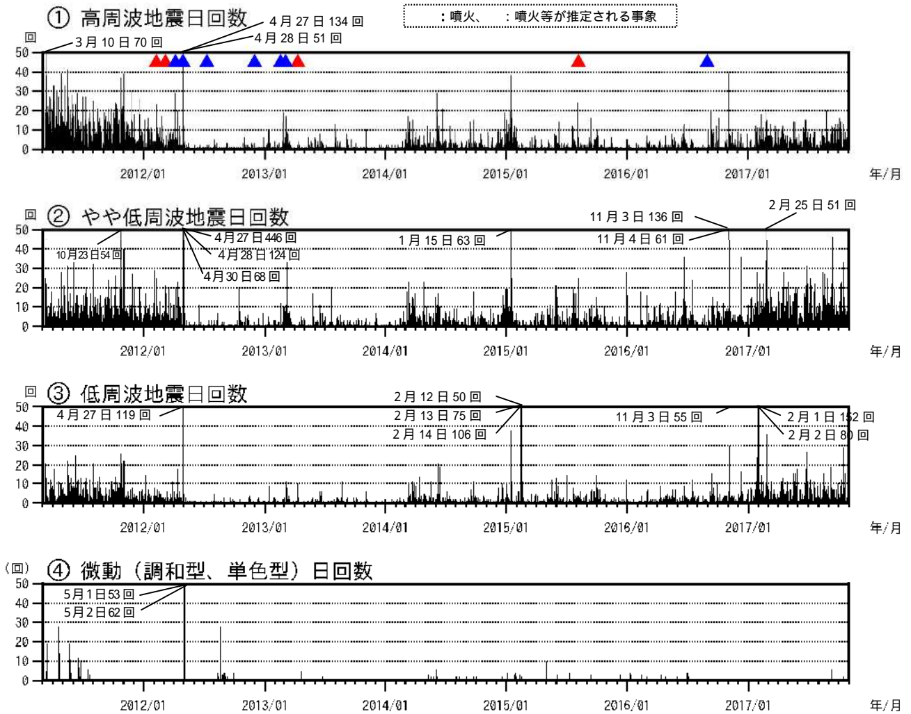
図4 硫黄島 火山活動経過図(2011年3月8日運用開始~2017年10月31日)
