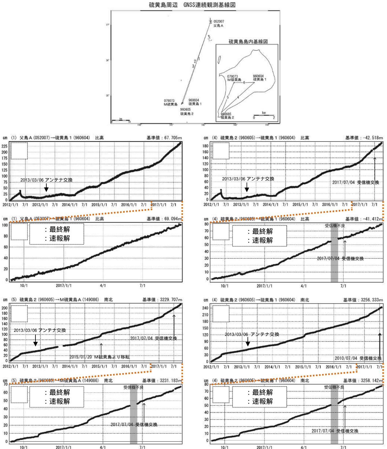
図5 硫黄島 国土地理院による地殻変動観測結果 2) ( 2012年1月1日~2017年9月26日、 2016年9月1日~2017年9月26日 ) のグラフ: 父島に対する硫黄島1の比高の変化 のグラフ: 硫黄島2(島西部の摺鉢山付近)に対する硫黄島1(島北部の元山地域)の比高の変化 のグラフ: 硫黄島2に対するM硫黄島(島西部の阿蘇台陥没孔付近)の南北の変化 のグラフ: 硫黄島2に対する硫黄島1の南北の変化
