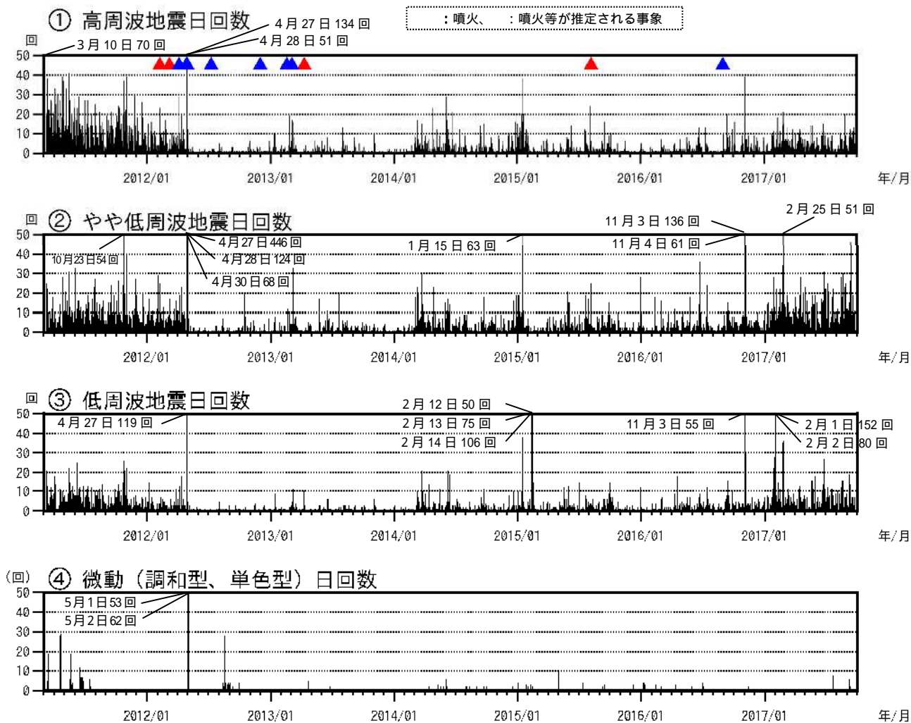
図4 硫黄島 火山活動経過図(2011年3月8日~2017年9月30日)
