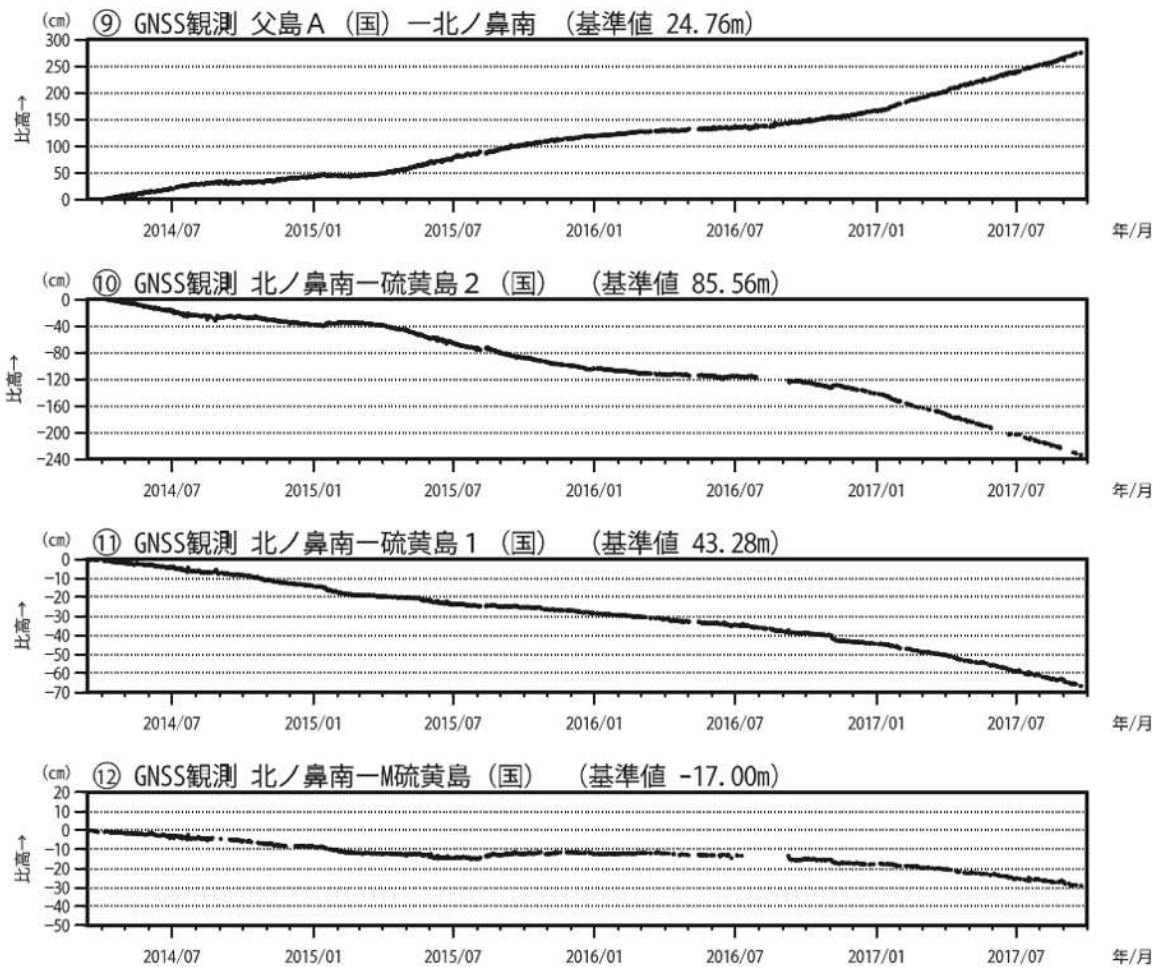
図6 硫黄島 GNSS 観測結果（2014年3月13日～2017年9月30日）（国）：国土地理院 ・基線 ~ は図7の ~ に対応します。いずれの図も、左の観測点に対する右の観測点の比高（高度の差）の変化を表しています。グラフの空白部分は欠測を示します。
