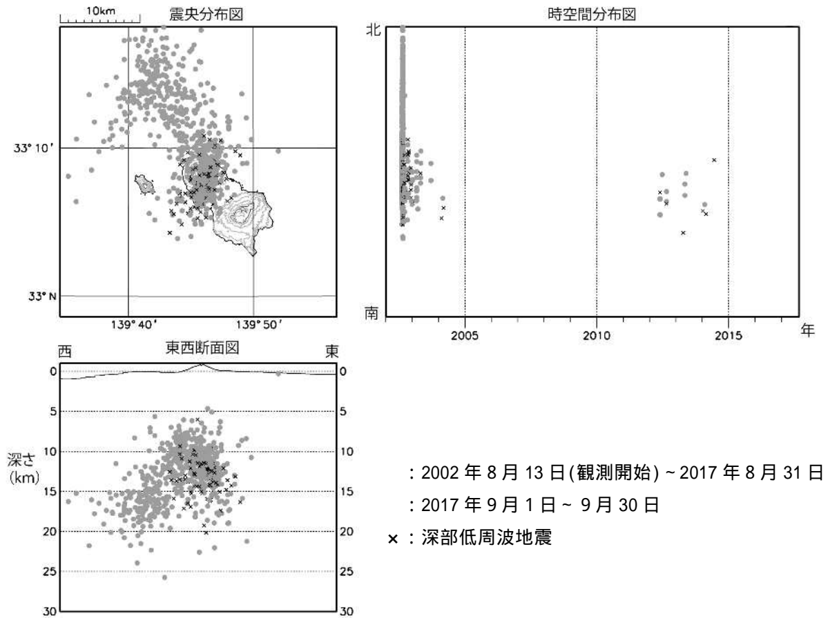
図3 八丈島 震源分布図（2002年8月13日～2017年9月30日） ・今期間、八丈島付近に震源が求まる高周波地震及び深部低周波地震はありませんでした。
