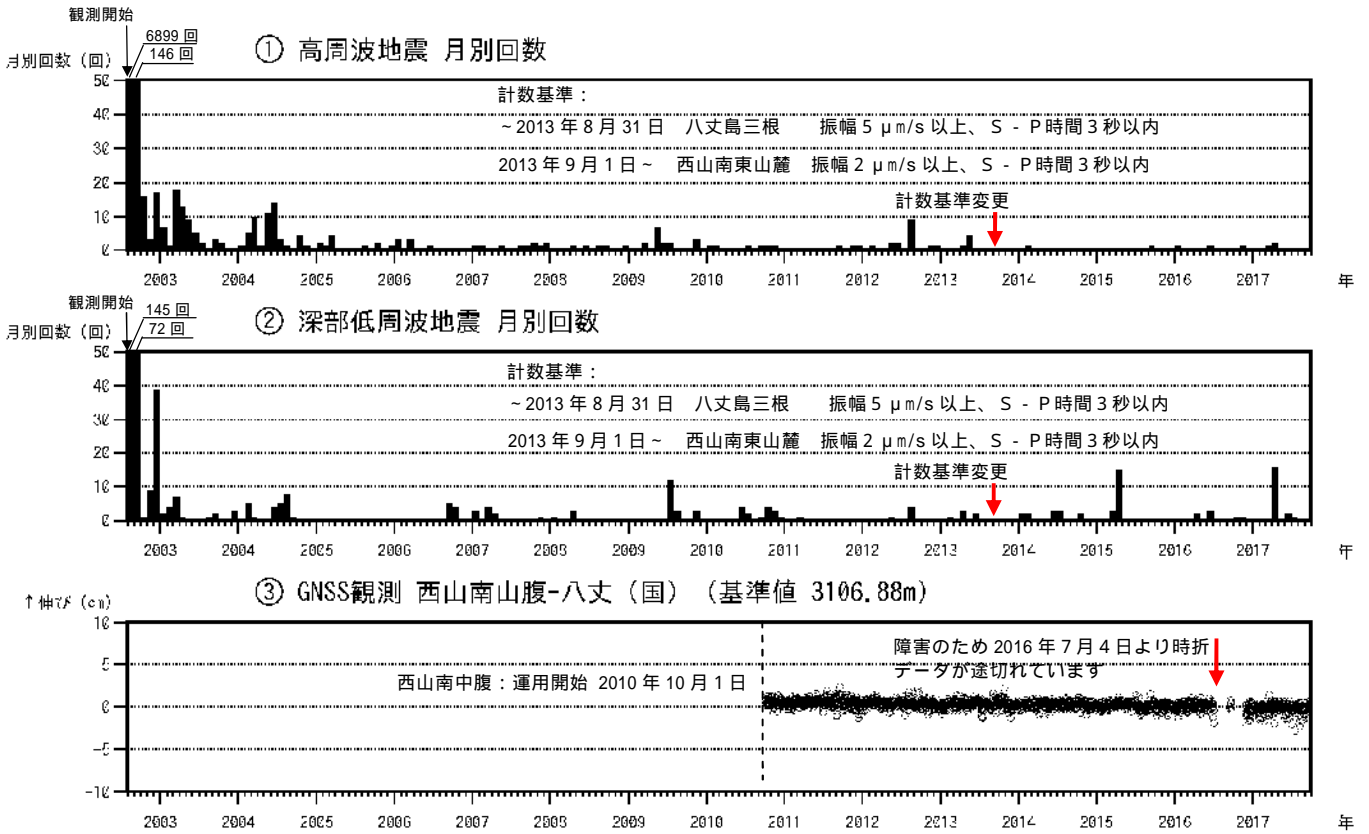
図2 八丈島 火山活動経過図(2002年8月13日~2017年9月30日)
