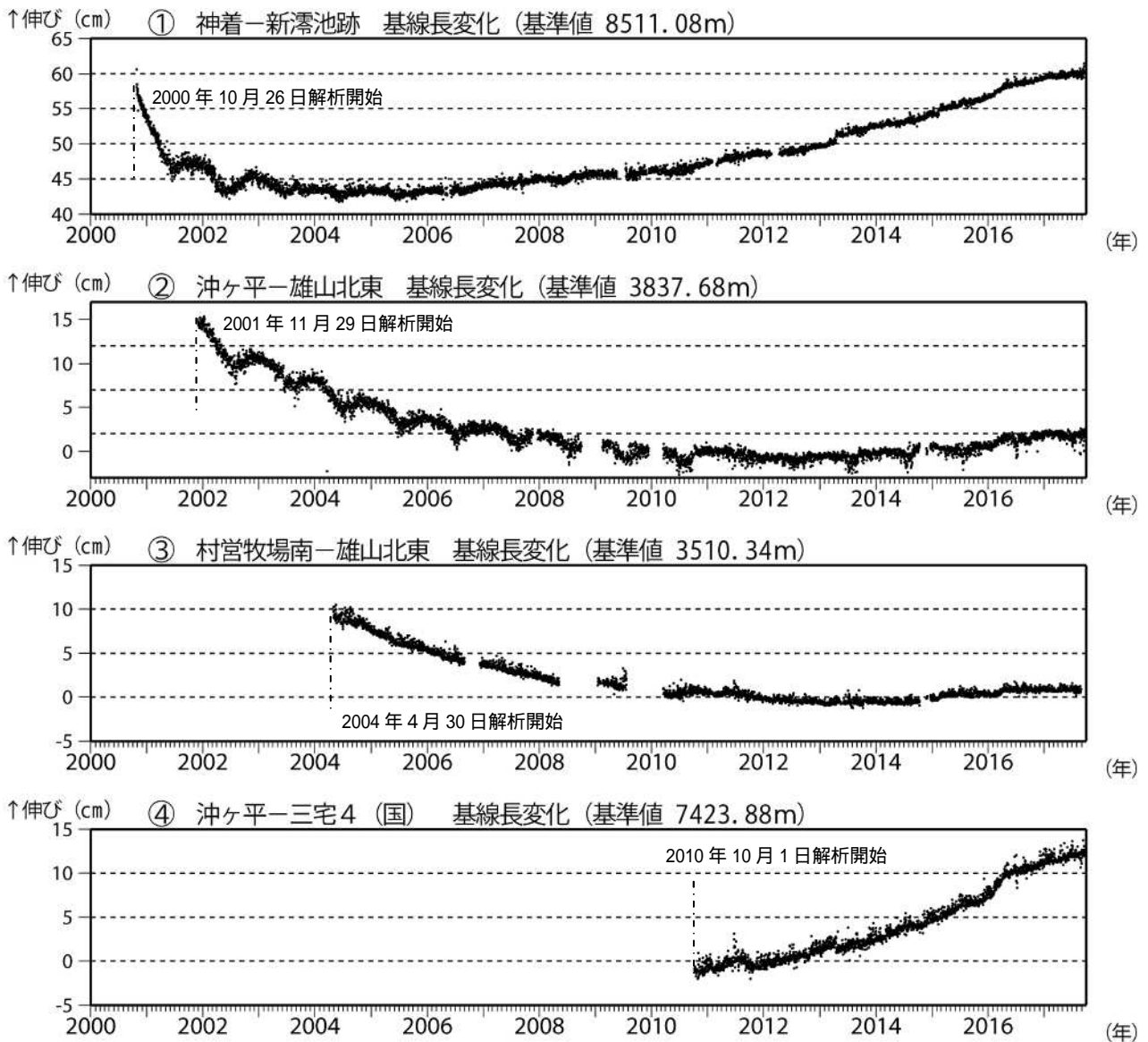
図7 三宅島 GNSS 連続観測結果 (2000年10月26日~2017年9月30日) (国): 国土地理院
