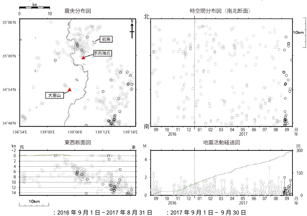
図2 伊豆東部火山群 広域地震観測網による震源分布図(2016年9月1日~2017年9月30日)
