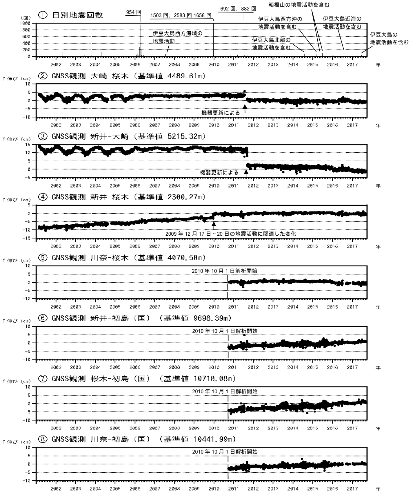
図3 伊豆東部火山群 火山活動経過図(2001年1月1日~2017年9月30日)
