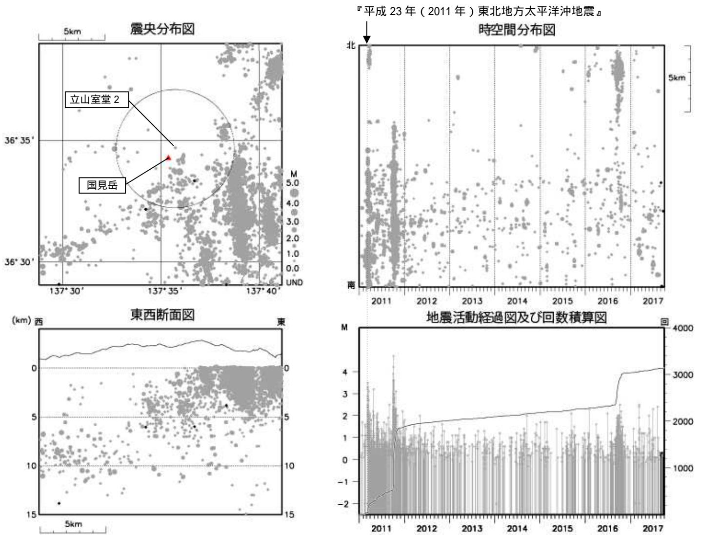
図 2 弥陀ヶ原 広域地震観測網による山体・周辺の地震活動（2011 年 1 月 1 日～2017 年 9 月 30 日） : 2011 年 1 月 1 日～2017 年 8 月 31 日 : 2017 年 9 月 1 日～9 月 30 日
