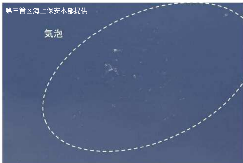
図 1 明神礁付近の気泡
