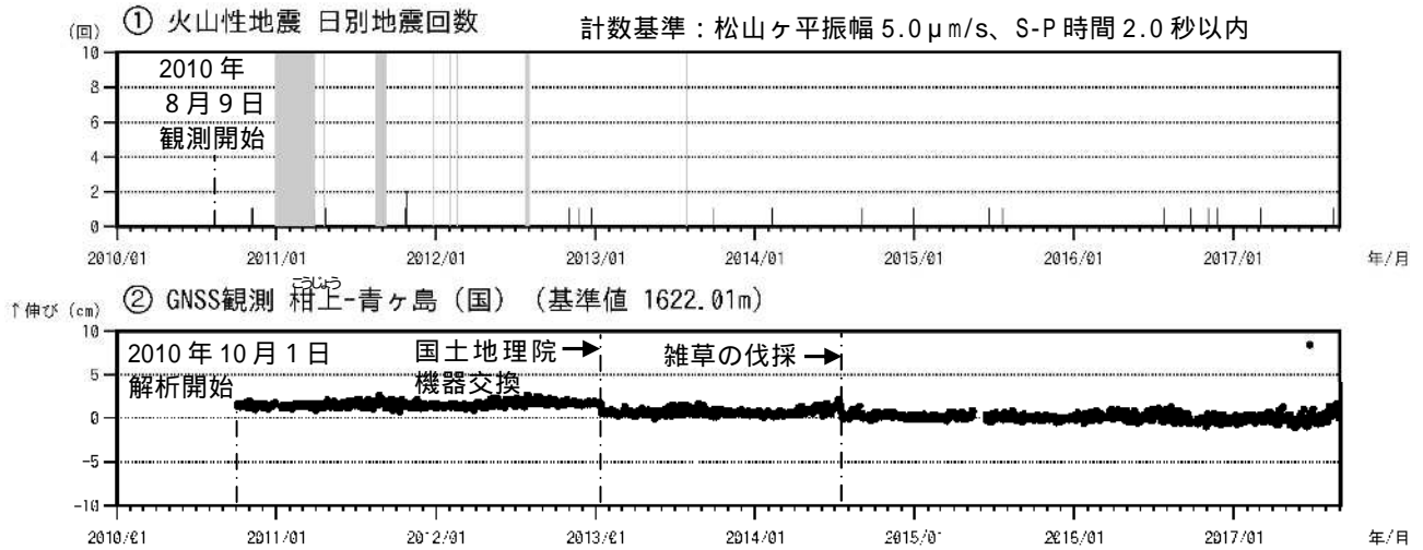
図2 青ヶ島 火山活動経過図（2010年8月9日～2017年8月31日） 青ヶ島周辺の日別地震回数 グラフの灰色部分は機器障害による欠測。 GNSS連続観測による基線長変化（国）：国土地理院 は図3のGNSS基線に対応。グラフの空白部分は欠測。 ・2014年7月15日に実施した雑草の伐採の影響により、ステップ状の変化がみられます。
