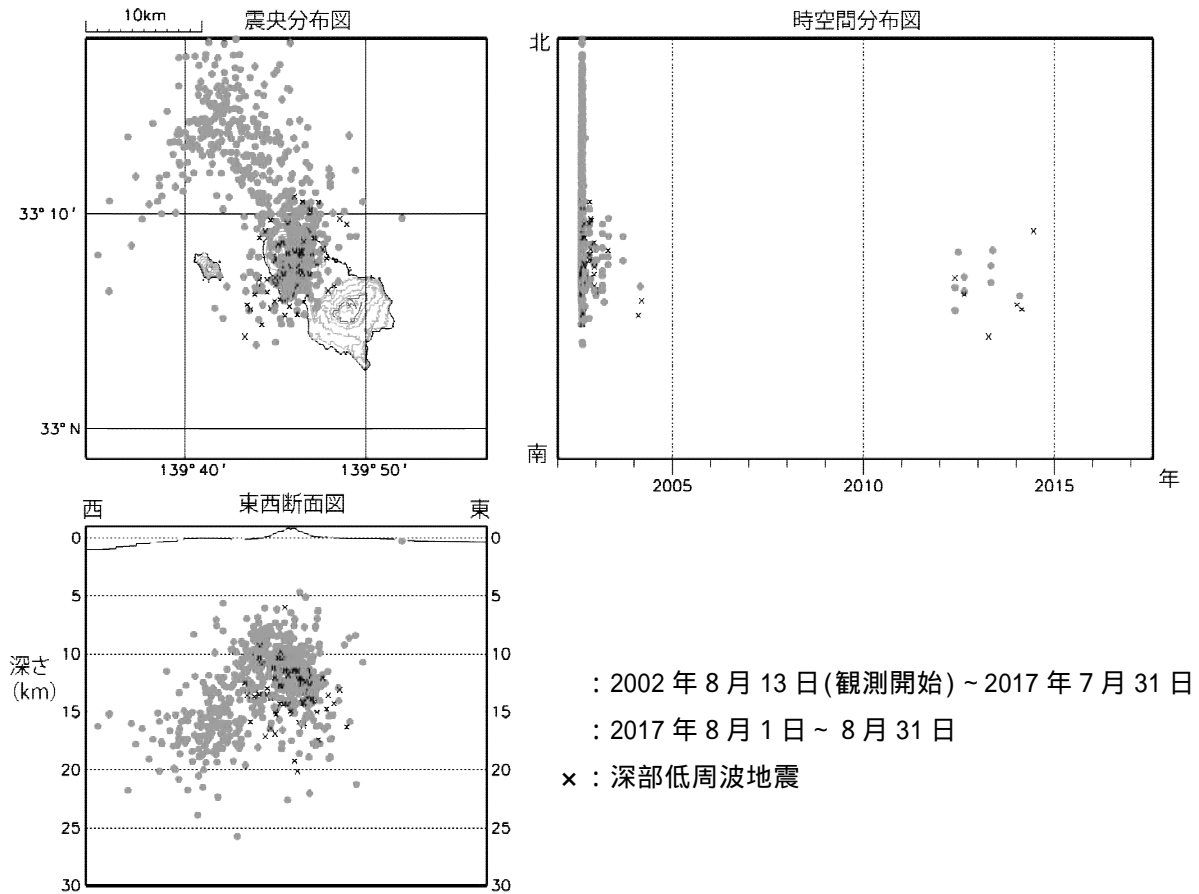
図3 八丈島 震源分布図（2002年8月13日～2017年8月31日） ・今期間、八丈島付近に震源が求まる高周波地震及び深部低周波地震はありませんでした。
