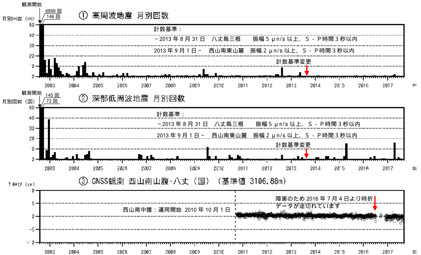
図2 八丈島 火山活動経過図（2002年8月13日～2017年8月31日）
