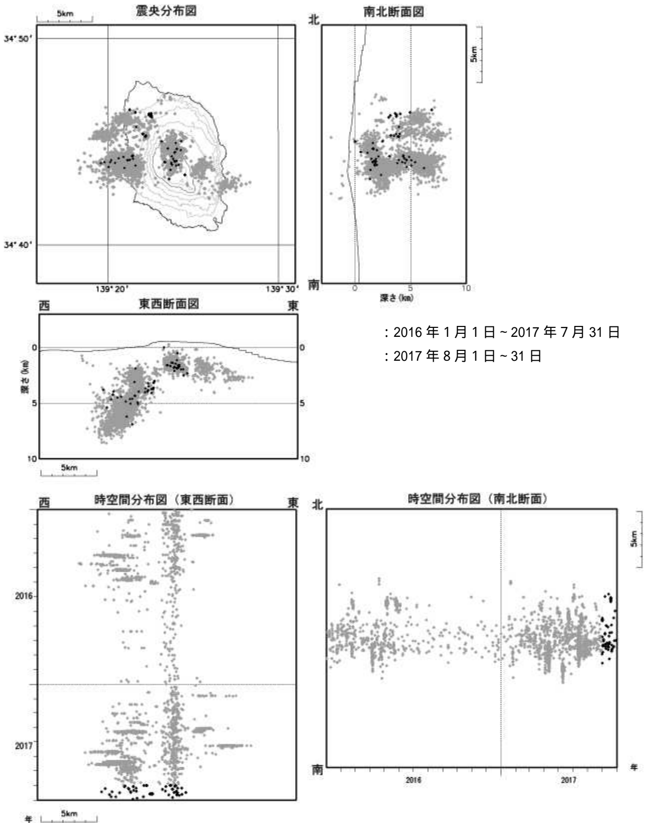
図4 伊豆大島 震源分布図(2016年1月1日~2017年8月31日)
