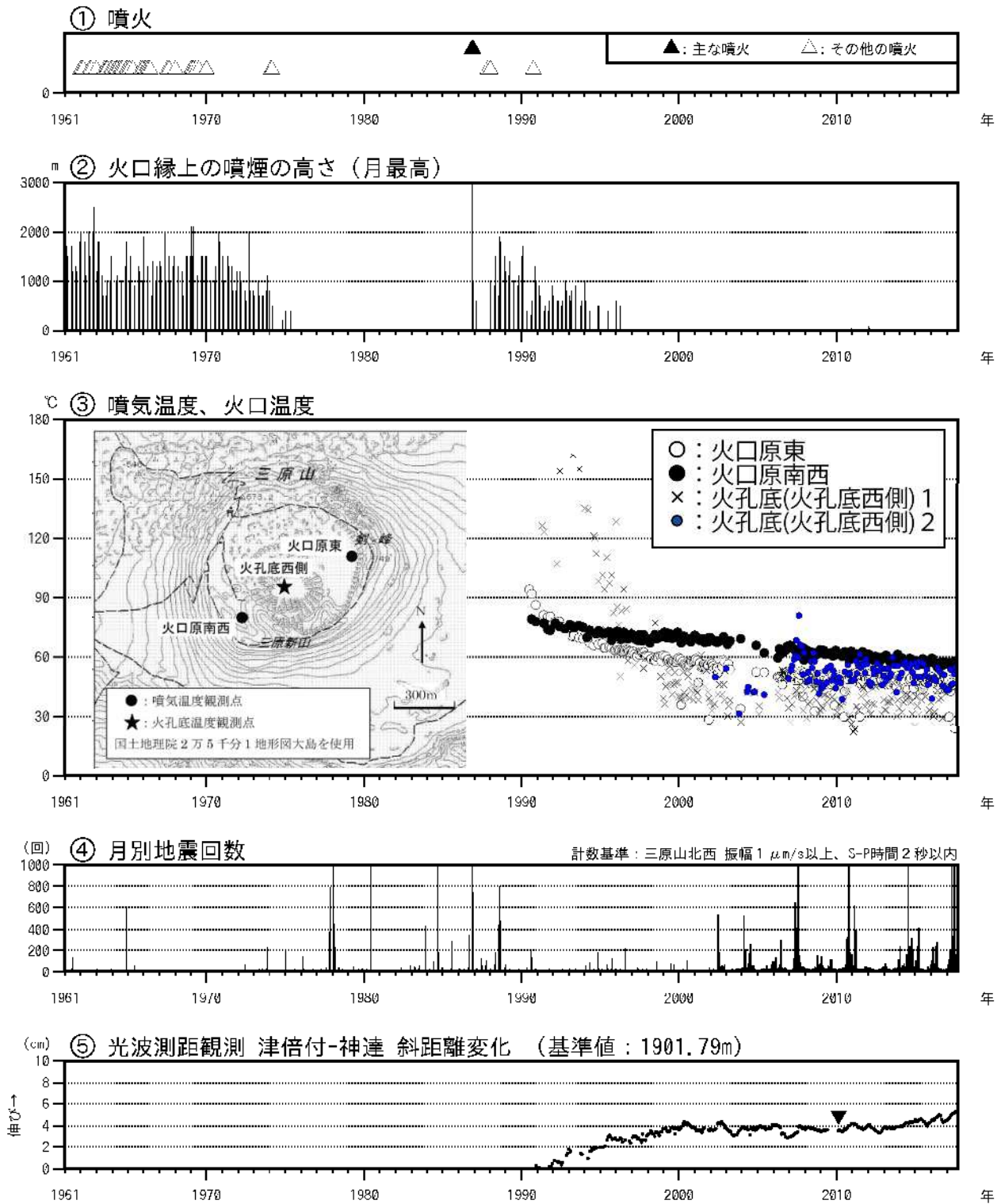
図1 伊豆大島 長期間の火山活動経過図(1961年1月~2017年8月31日)
