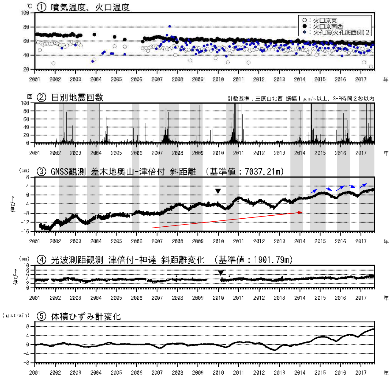
図 2 伊豆大島 最近の火山活動経過図（2001 年 1 月～2017 年 8 月 31 日）
