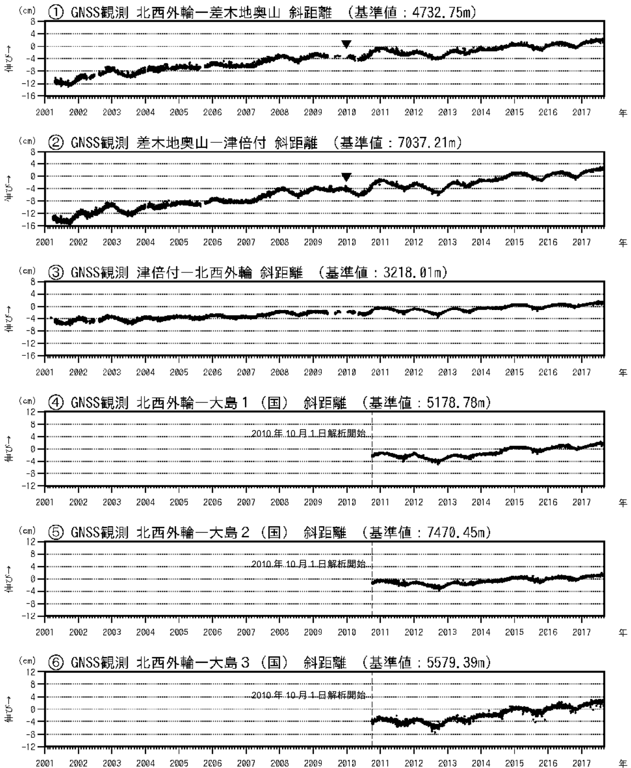
図3 伊豆大島 GNSS 連続観測による基線長変化(2001 年 1 月～2017 年 8 月 31 日)
