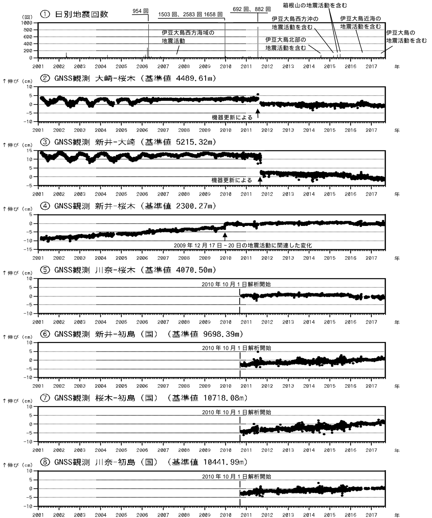
図3 伊豆東部火山群 火山活動経過図(2001年1月1日~2017年8月31日)
