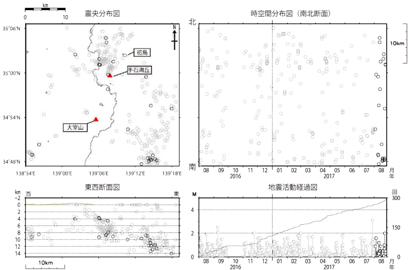
図2 伊豆東部火山群 広域地震観測網による震源分布図(2016年8月1日～2017年8月31日)
