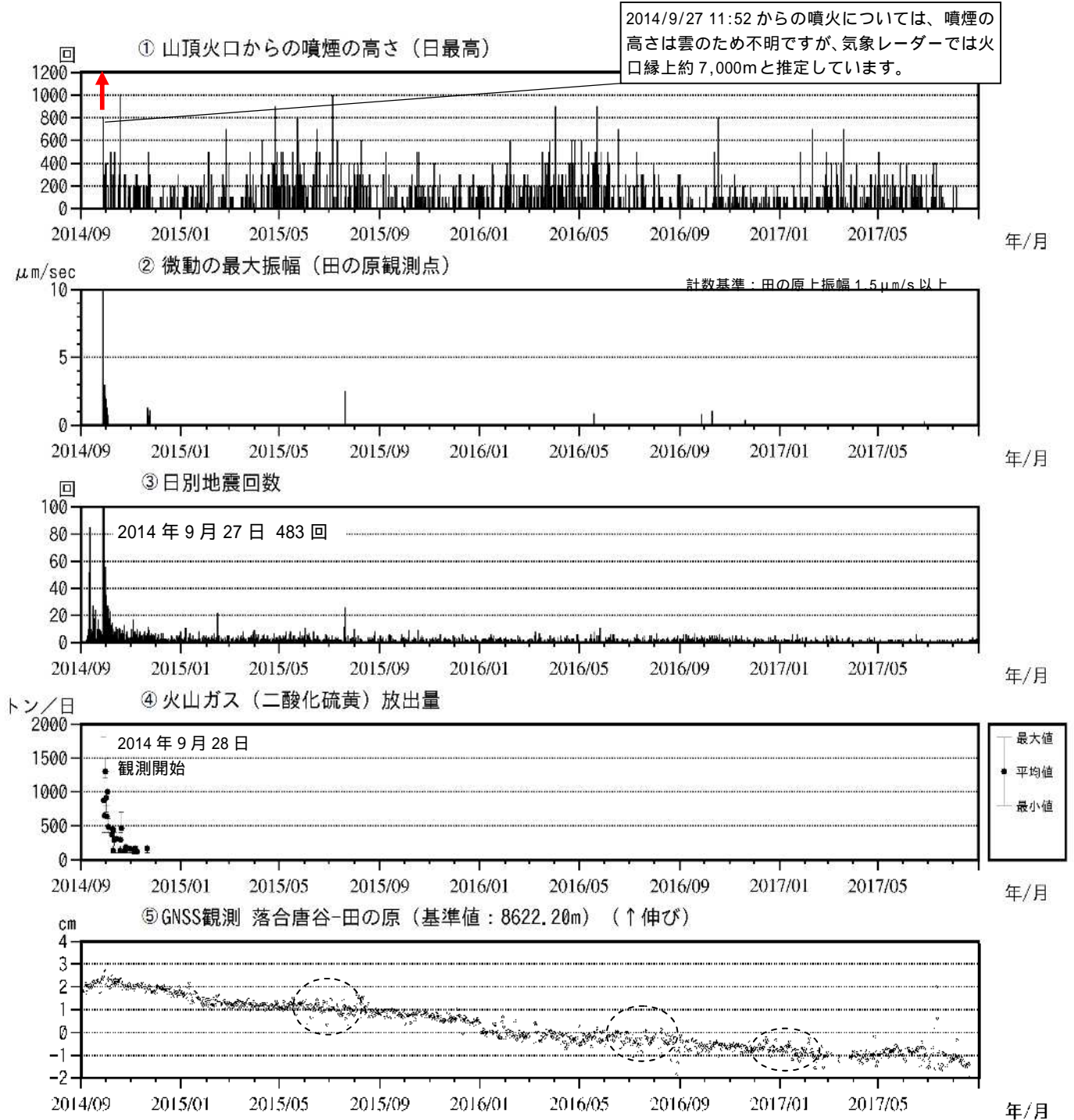
図3 御嶽山 最近の火山活動経過図 (2014年9月1日~2017年8月31日)
