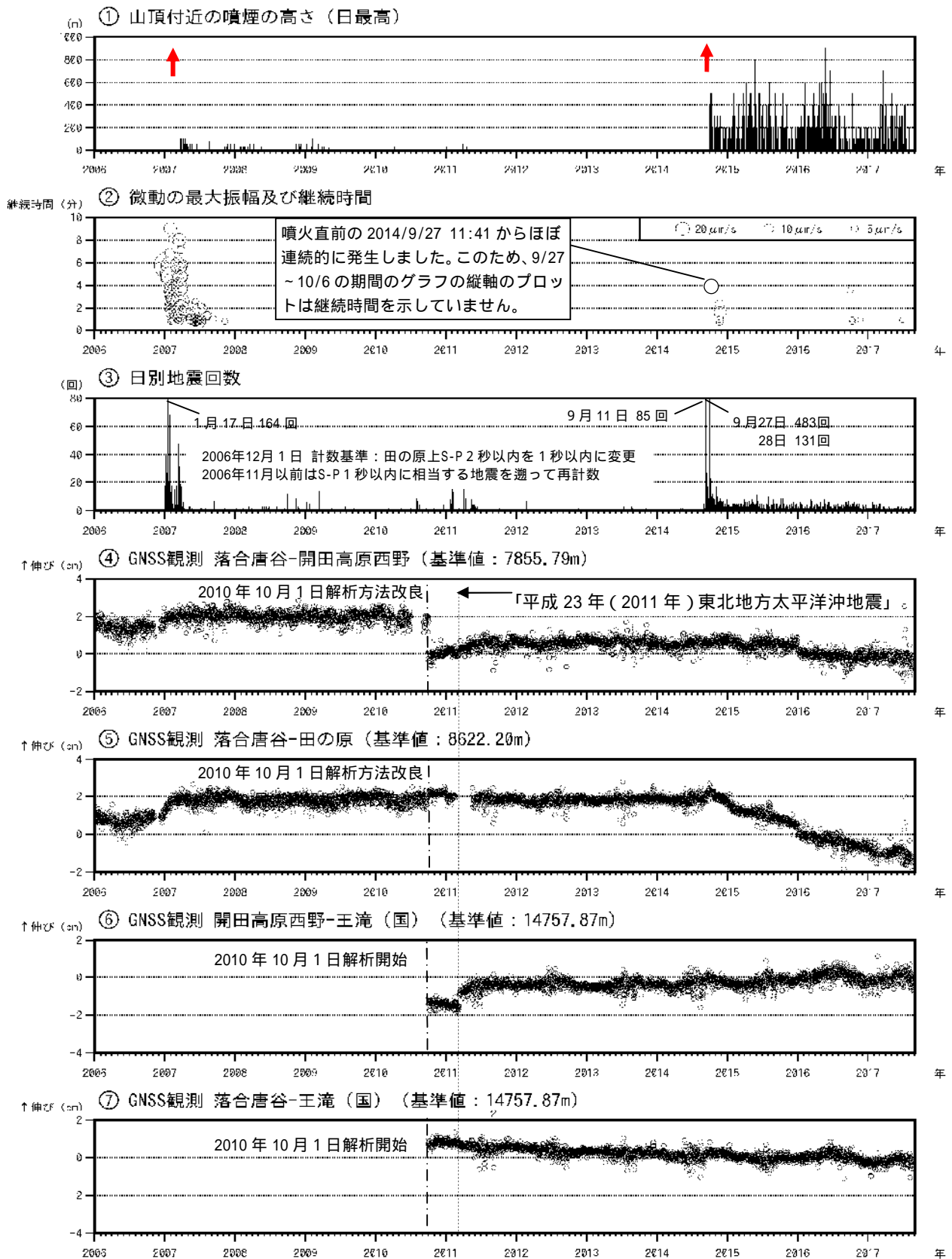
図4 御嶽山 長期間の火山活動経過図（2006年1月1日～2017年8月31日）
