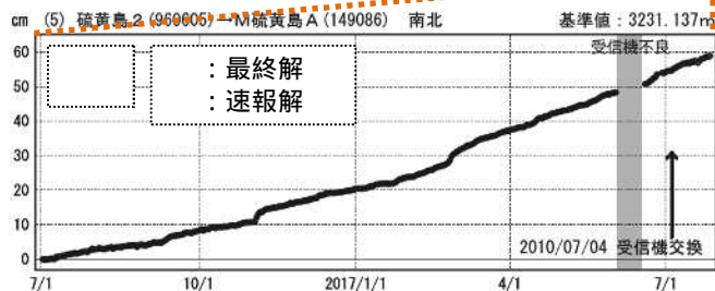
図 5 硫黄島 国土地理院による地殻変動観測結果 2)
