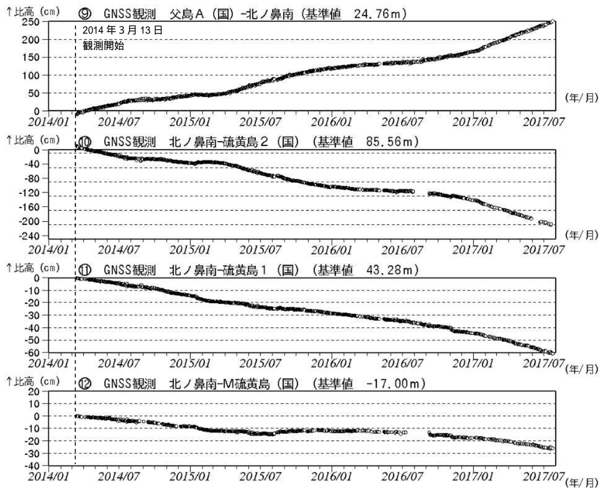
図6 硫黄島 GNSS 観測結果(2014年3月13日~2017年7月31日) (国): 国土地理院
