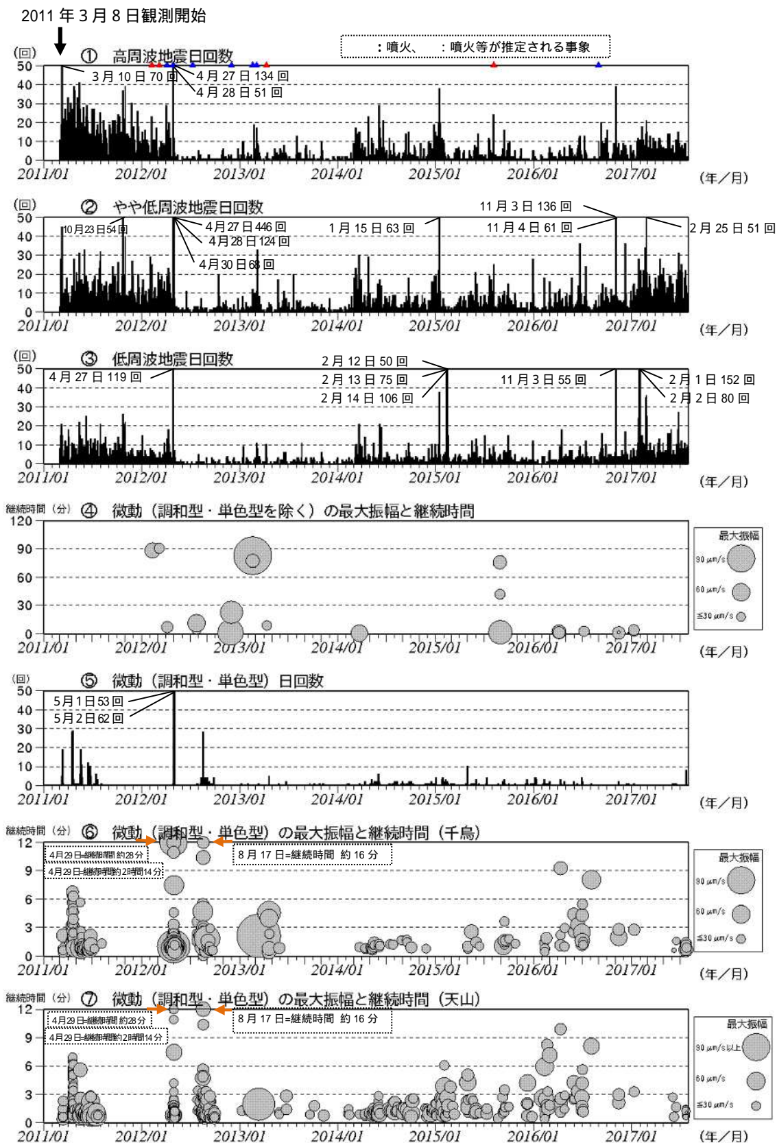
図4 硫黄島 火山活動経過図（2011年3月8日～2017年7月31日）
