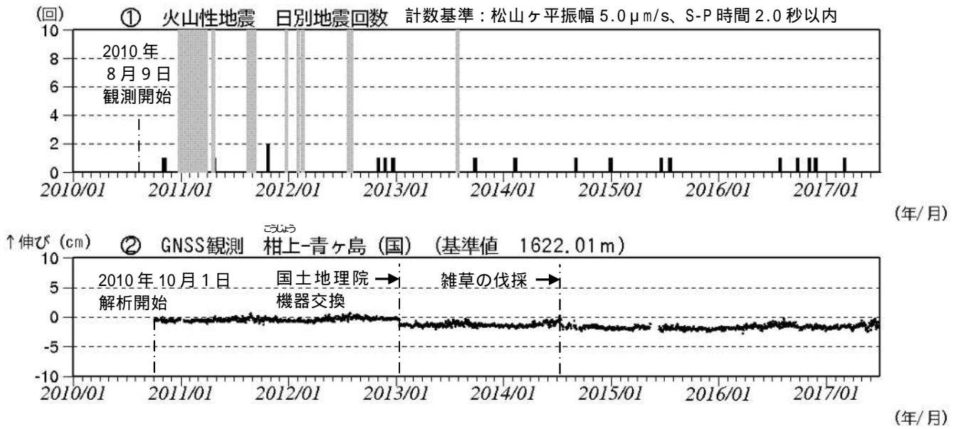
図2 青ヶ島 火山活動経過図(2010年8月9日~2017年6月30日) 青ヶ島周辺の日別地震回数 グラフの灰色部分は機器障害による欠測。 GNSS連続観測による基線長変化(国): 国土地理院 は図3のGNSS基線に対応。グラフの空白部分は欠測。 ・2014年7月15日に実施した雑草の伐採の影響により、ステップ状の変化がみられます。
