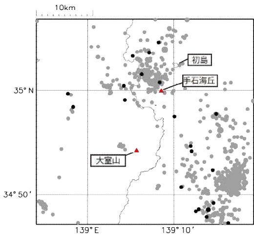
震央分布図
